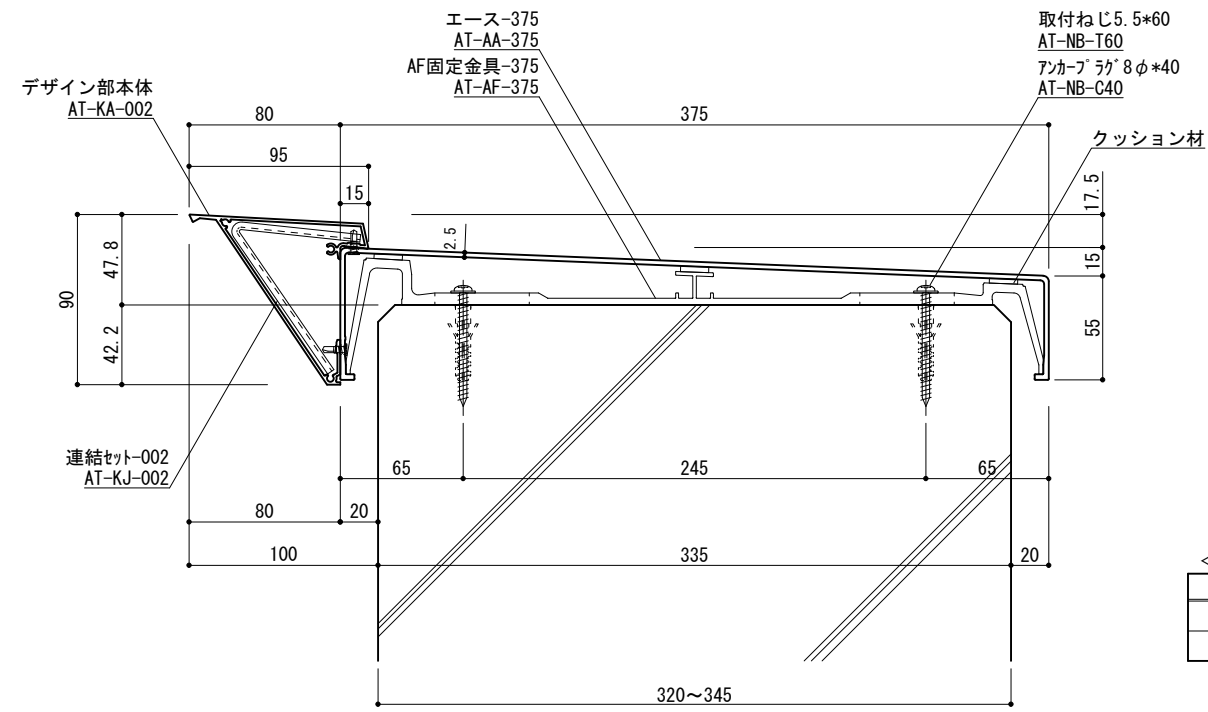
断面図 1/4
