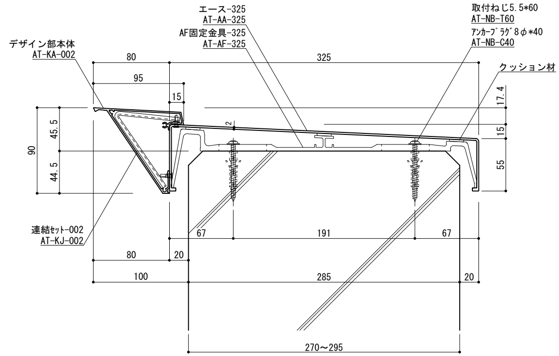
断面図 1/4
