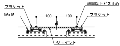
ジョイント部断面図
