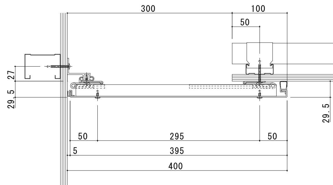
300-TCE 断面图
