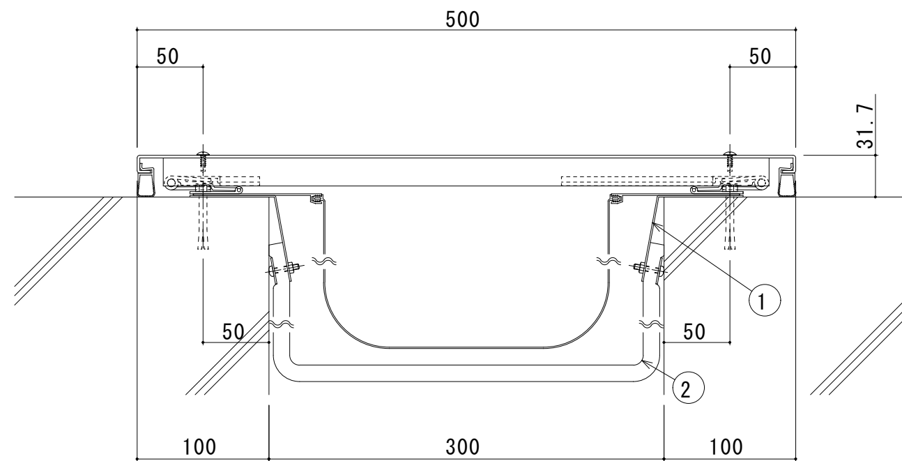
300-EE (遮炎仕様) 断面図
