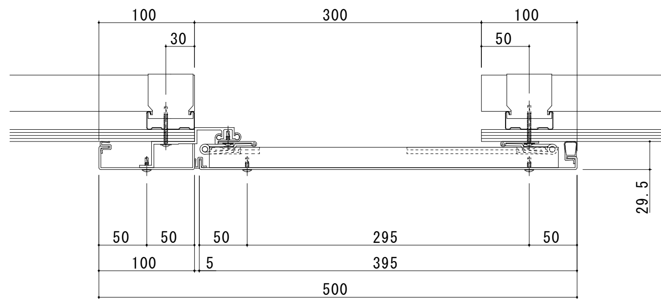
300-TE 断面图
