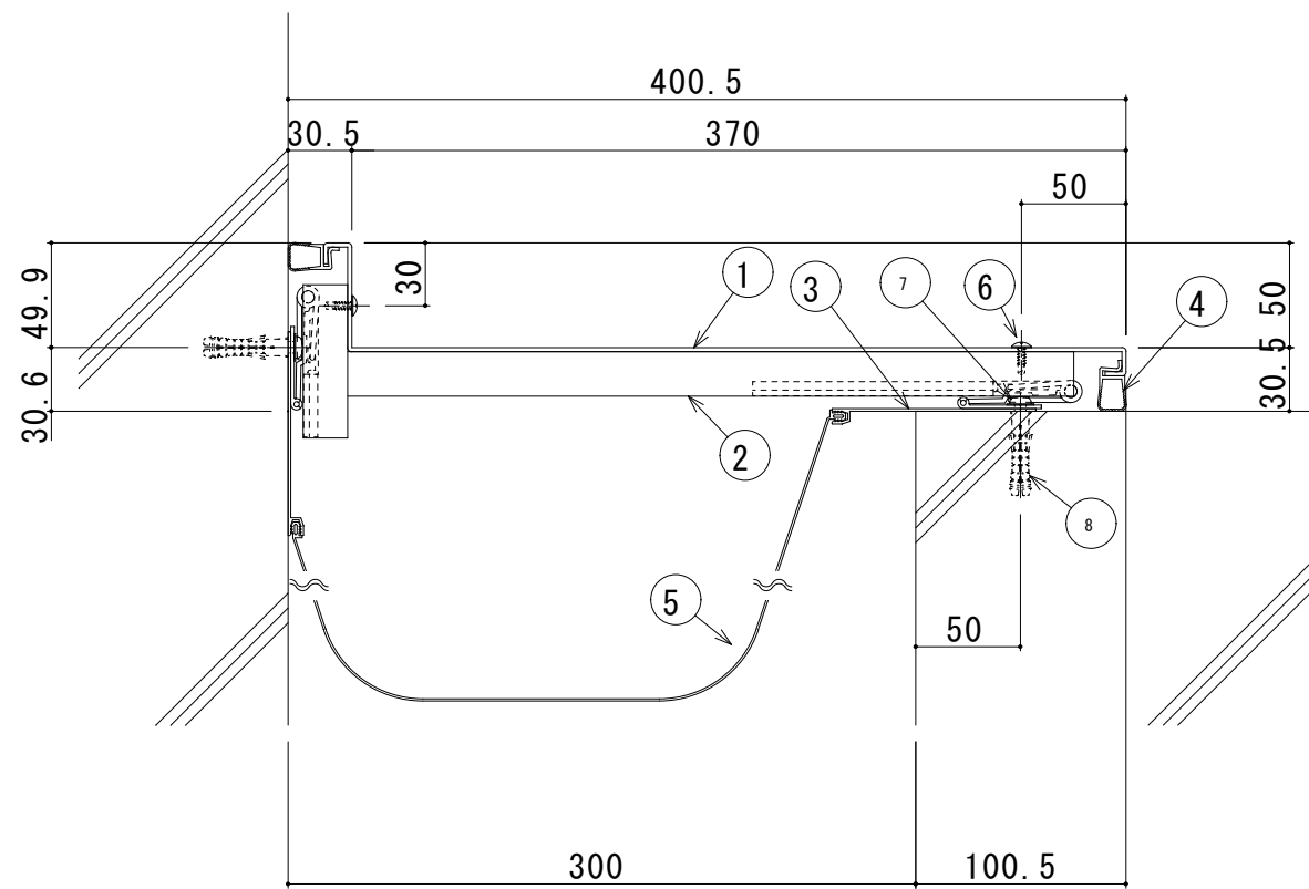
300-ECE 断面図
