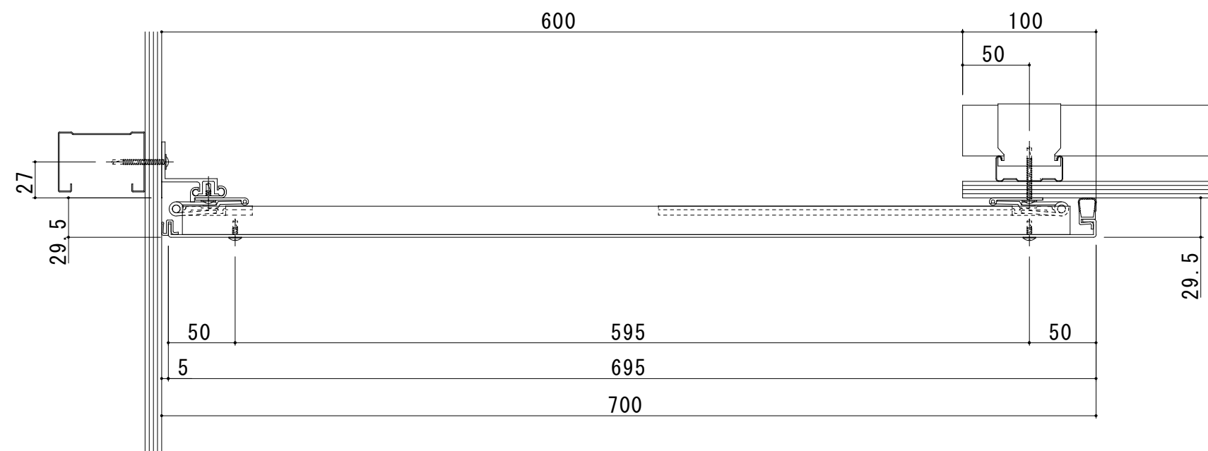
600-TCE 断面图
