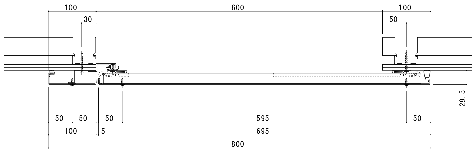
600-TE 断面图
