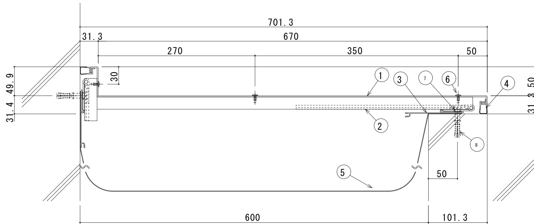
600-ECE 断面図
