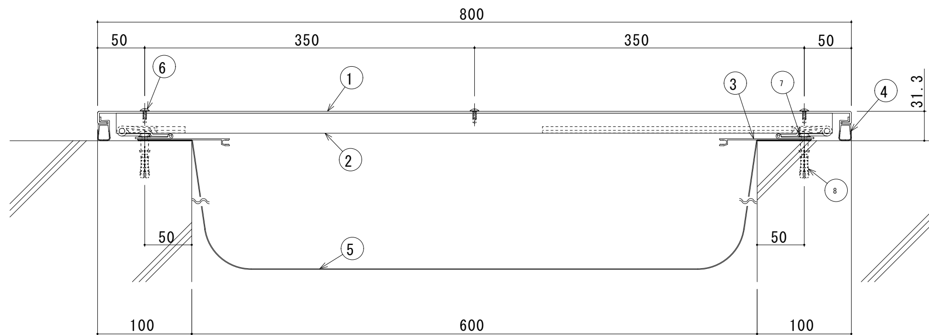
600-EE 断面図
