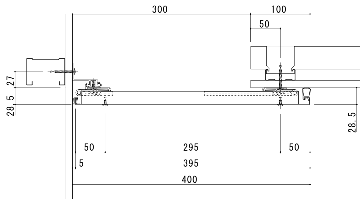
S300-TCE 断面图
