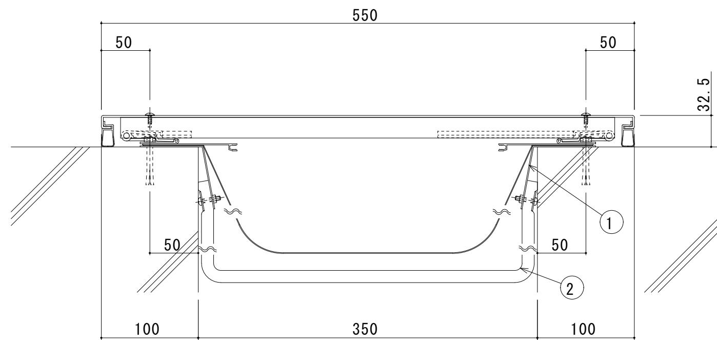
350-EE (遮炎仕様) 断面図
