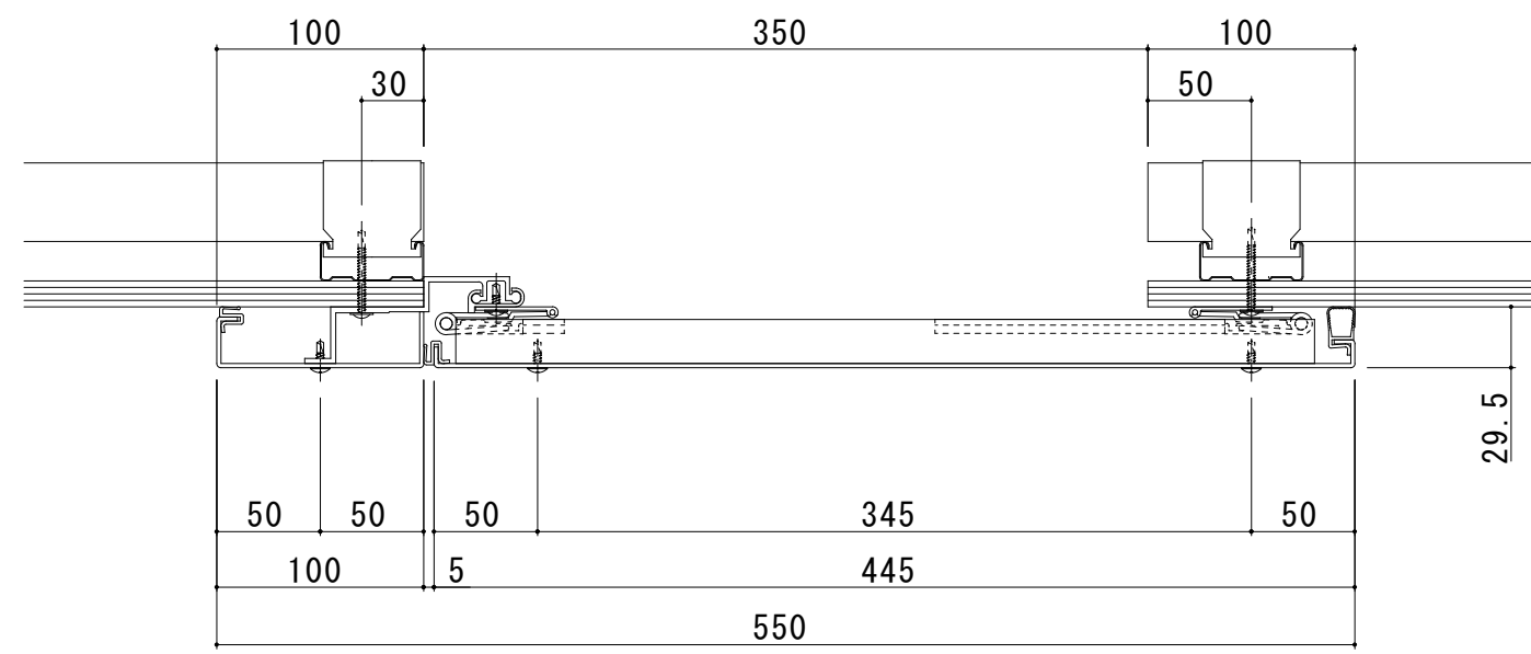
350-TE 断面图
