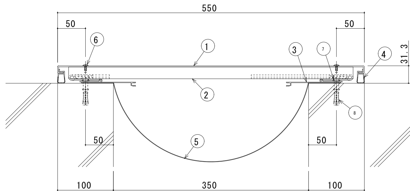
350-EE 断面図
