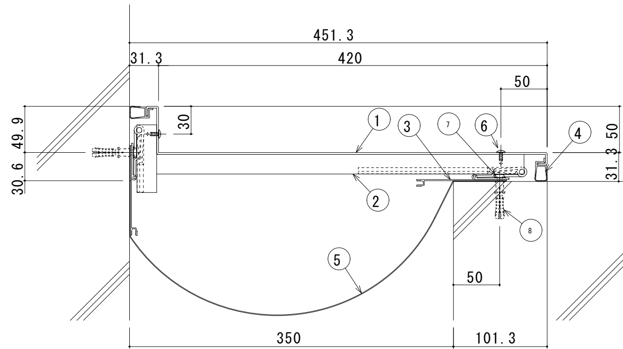
350-ECE 断面図
