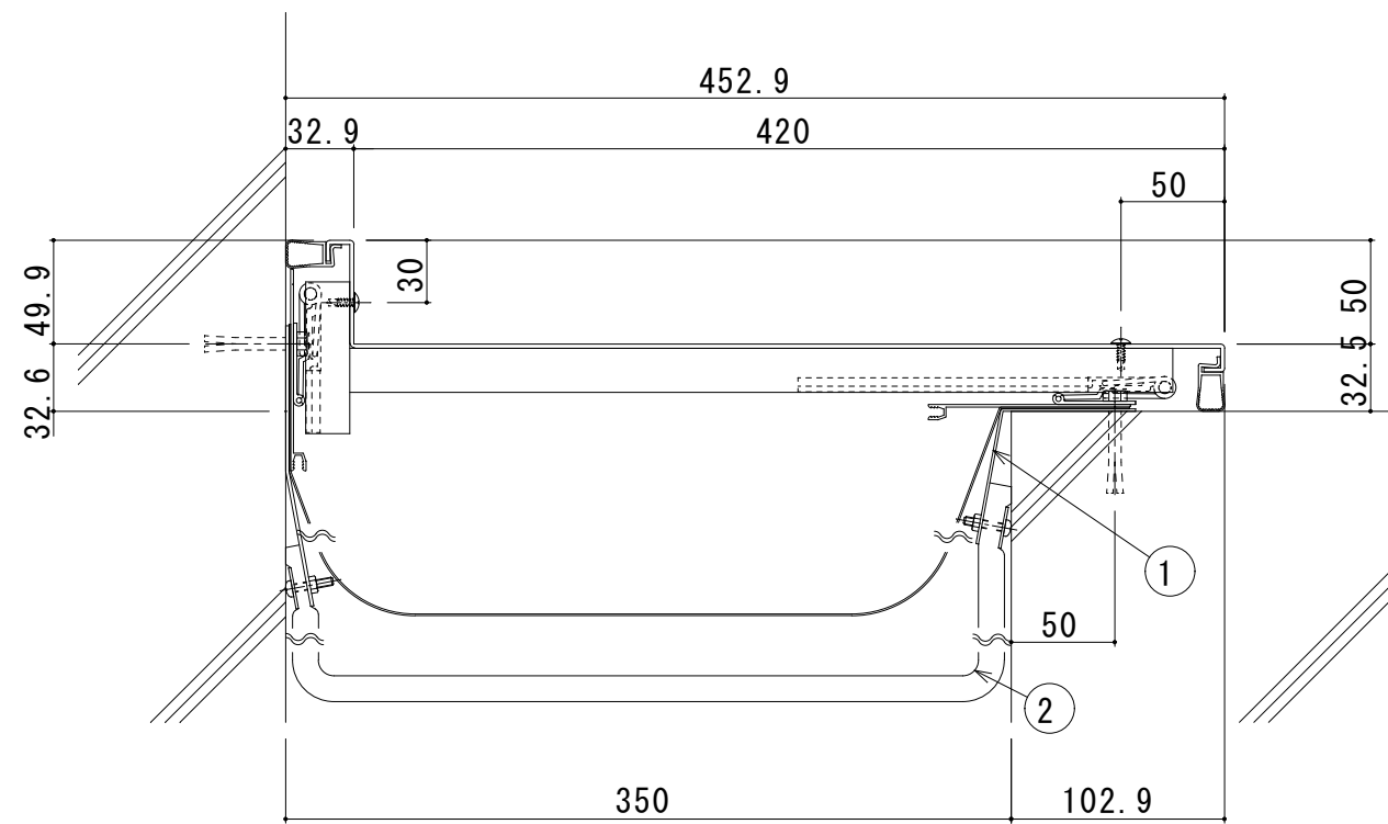
350-ECE (遮炎仕様) 断面図
