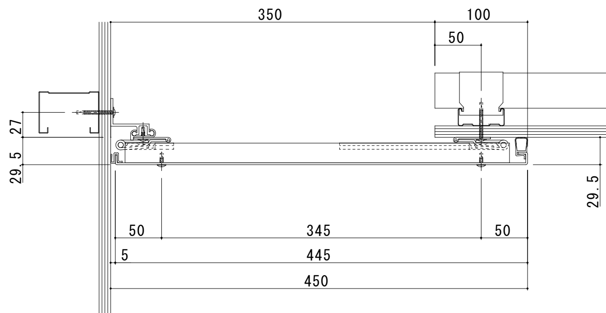
350-TCE 断面图
