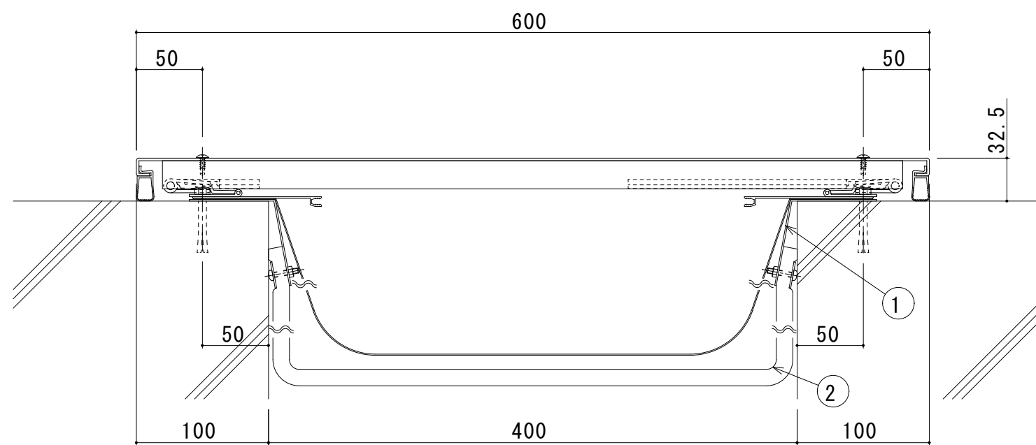
400-EE (遮炎仕様) 断面図
