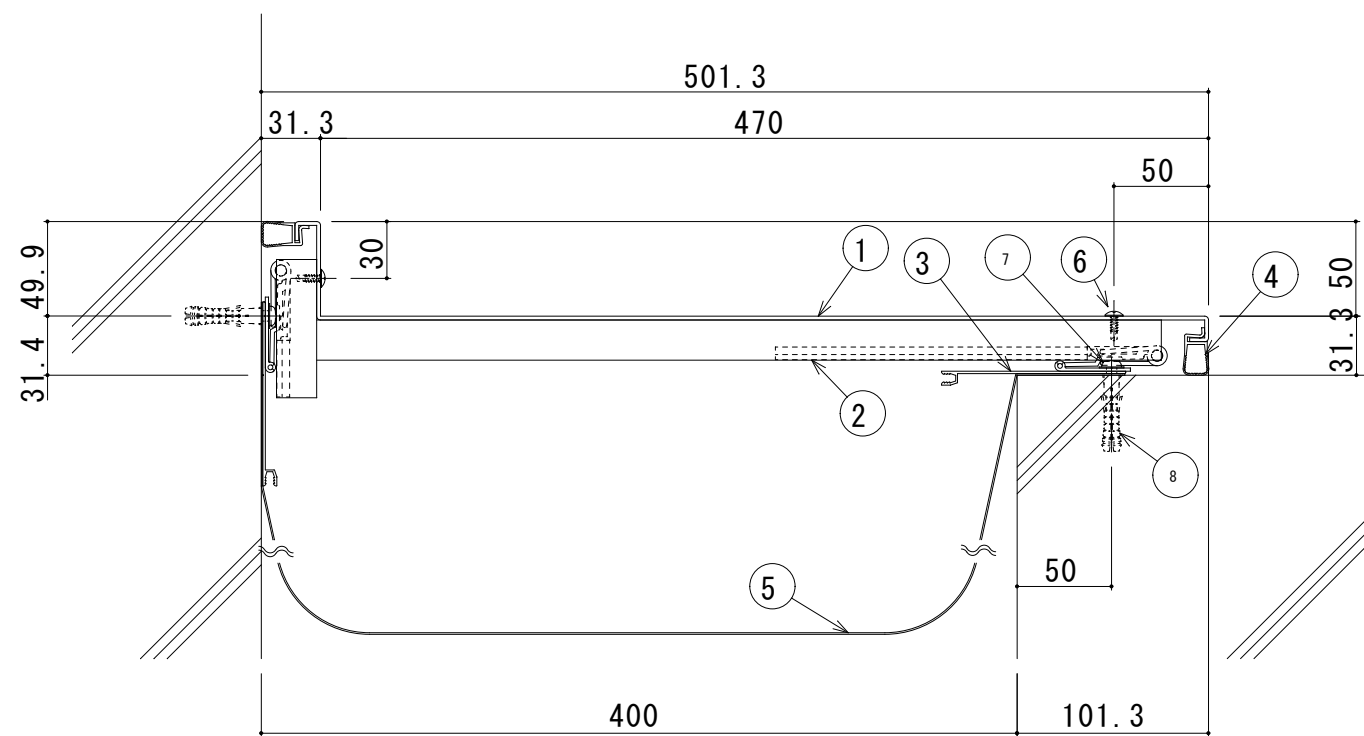
400-ECE 断面図
