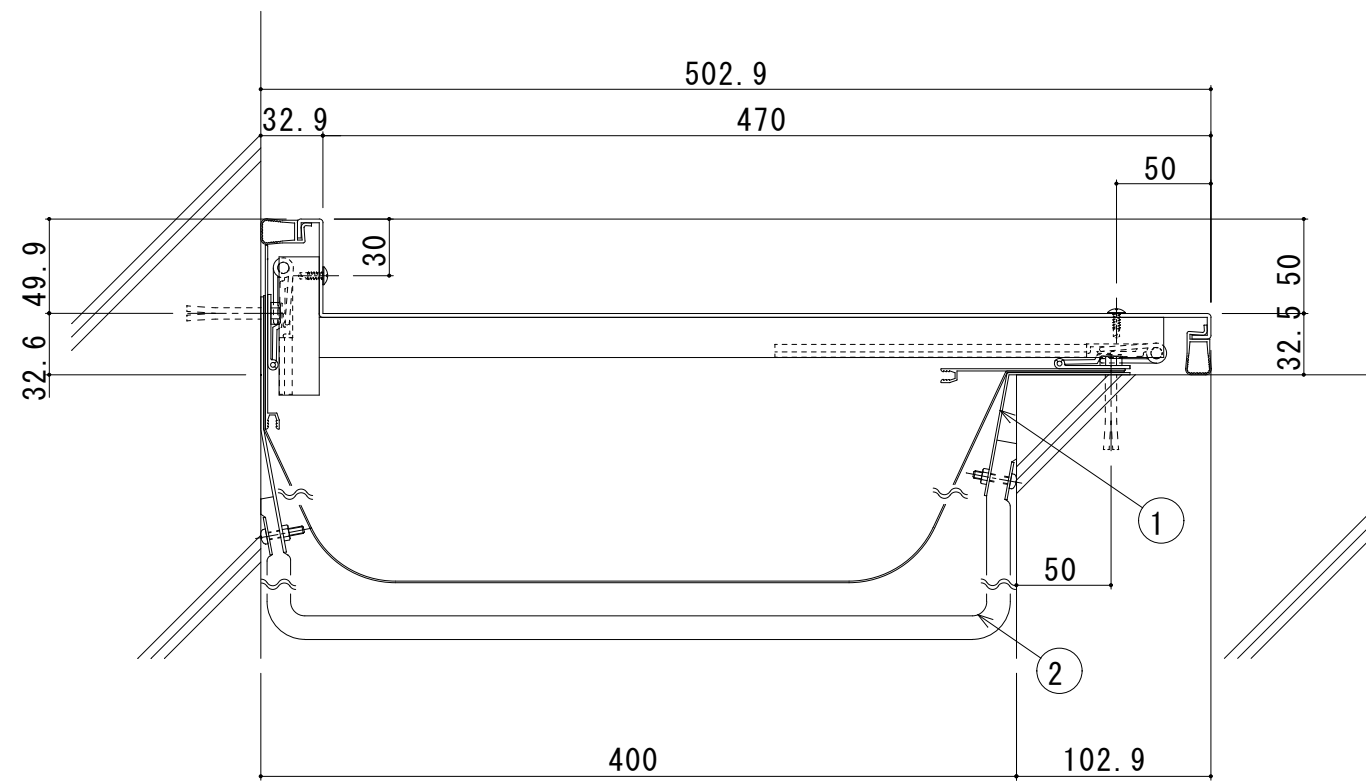
400-ECE (遮炎仕様) 断面図
