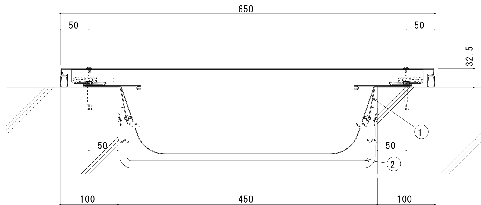
450-EE (遮炎仕様) 断面図
