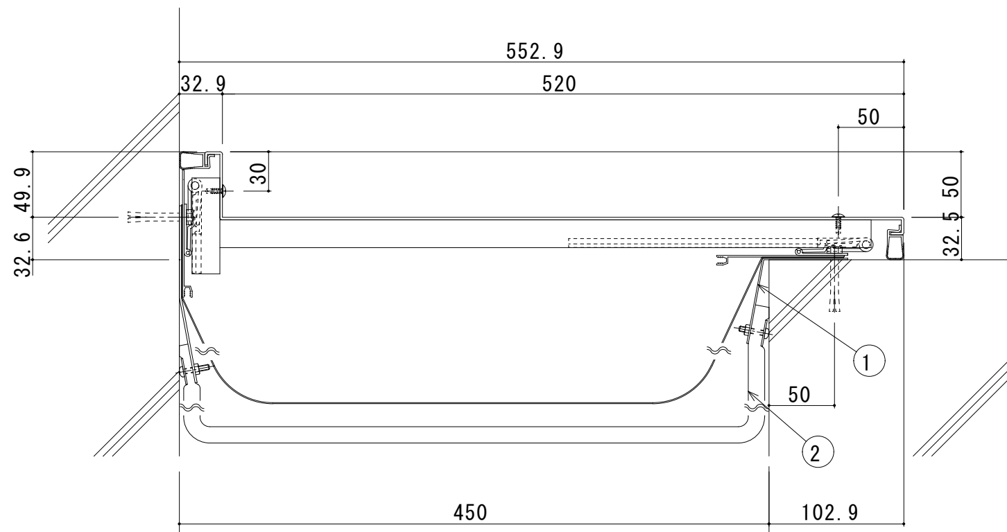
450-ECE (遮炎仕様) 断面図
