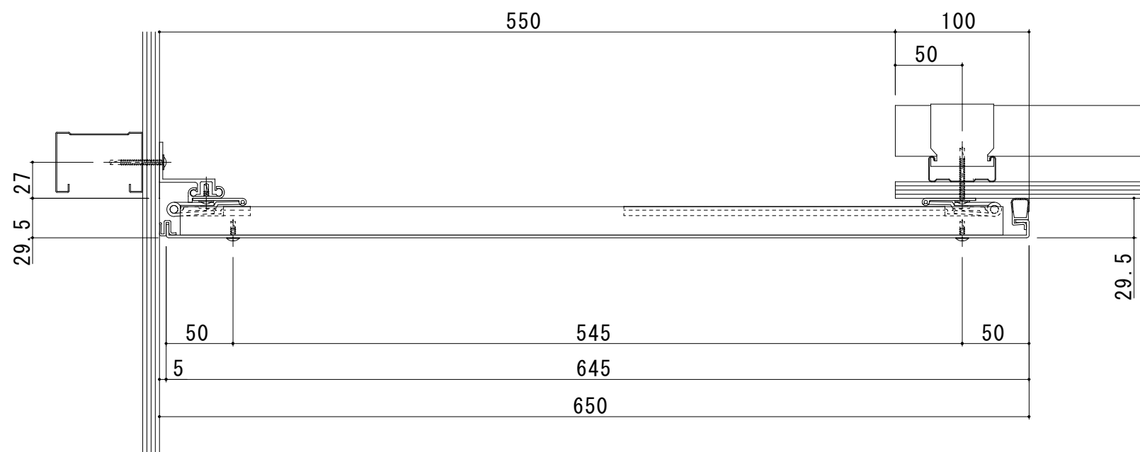
550-TCE 断面图
