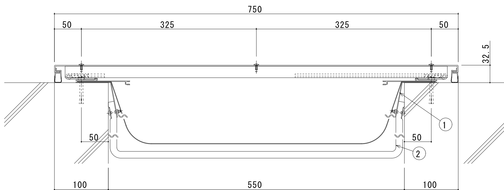
550-EE (遮炎仕様) 断面図
