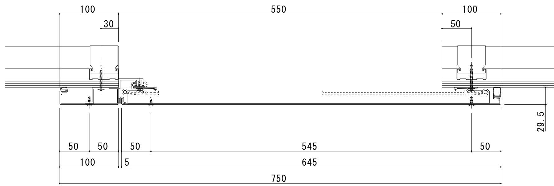
550-TE 断面图
