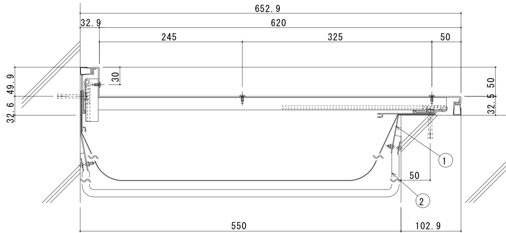
550-ECE (遮炎仕様) 断面図
