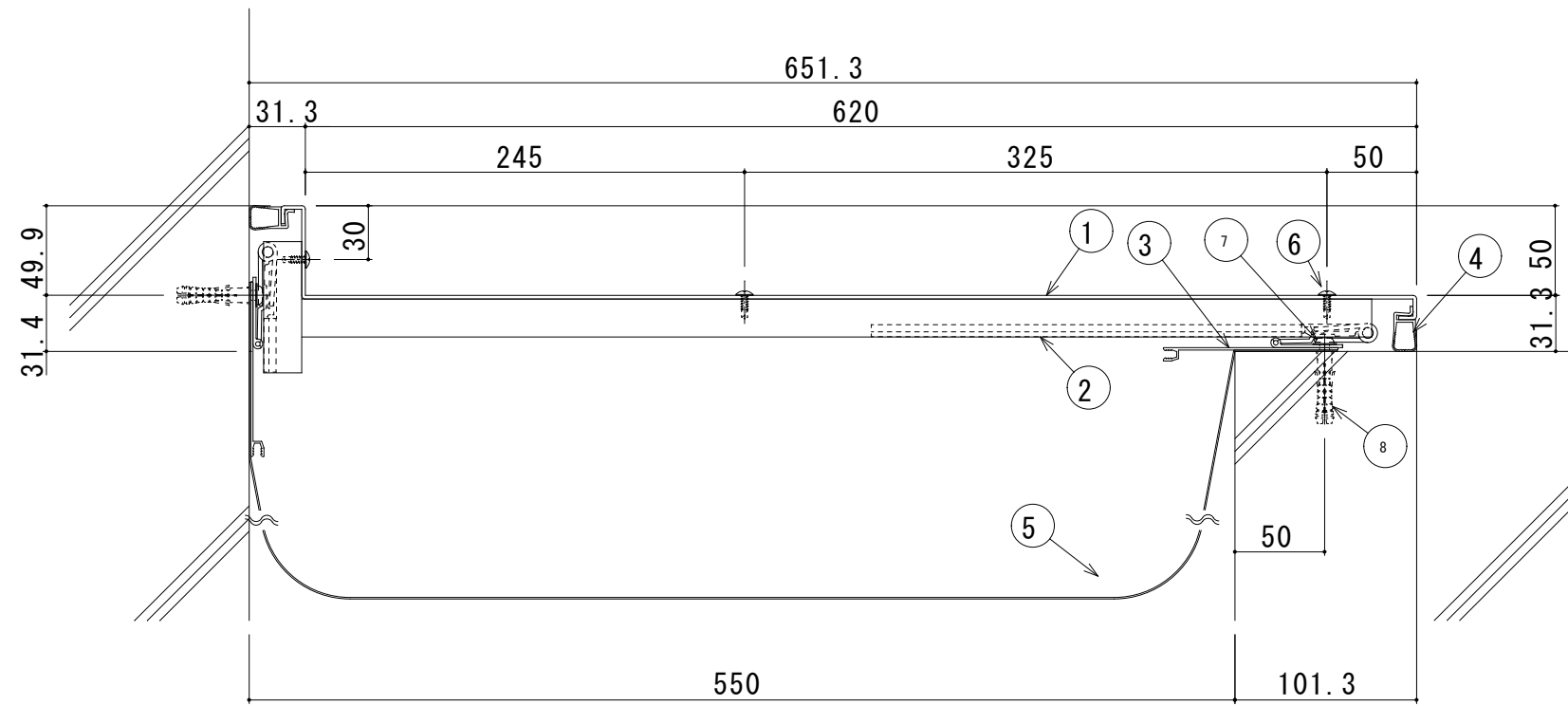
550-ECE 断面図
