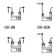
【100mm用 耐火帯】
