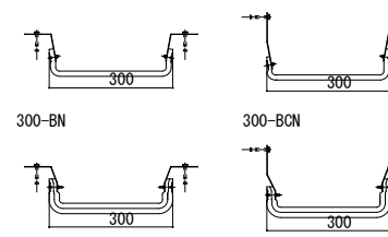
【300mm用 耐火帯】
