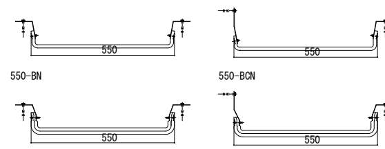
【550mm用 耐火帯】
