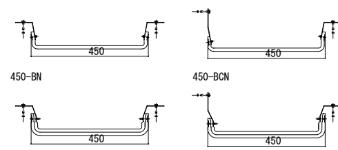
【450mm用 耐火帯】
