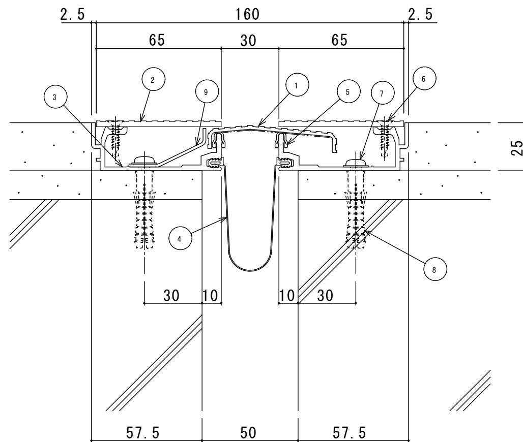
S50-FHJ-AS 断面図
