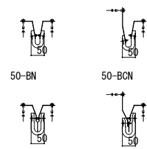
【50mm用 耐火帯】
