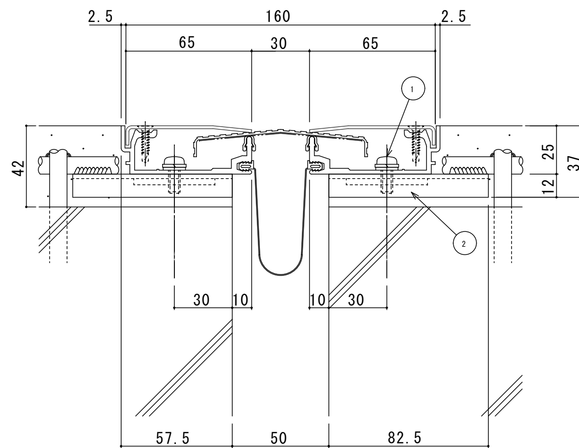
S50-FHA 断面図
