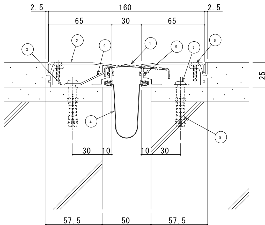
S50-FH-AS 断面図
