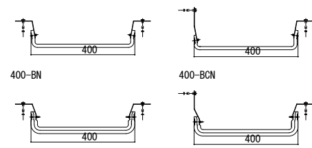
【400mm用 耐火帯】
