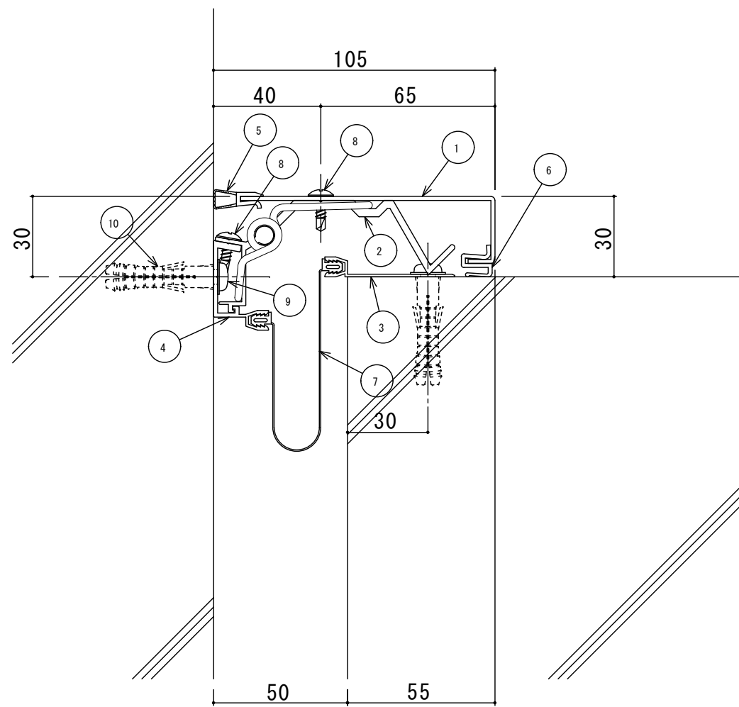
S50-ECH 断面図
