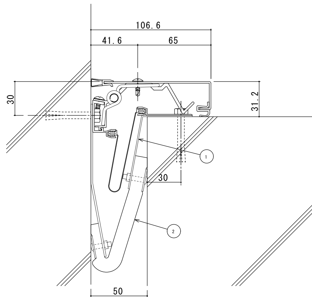
S50-ECH（遮炎仕様） 断面図
