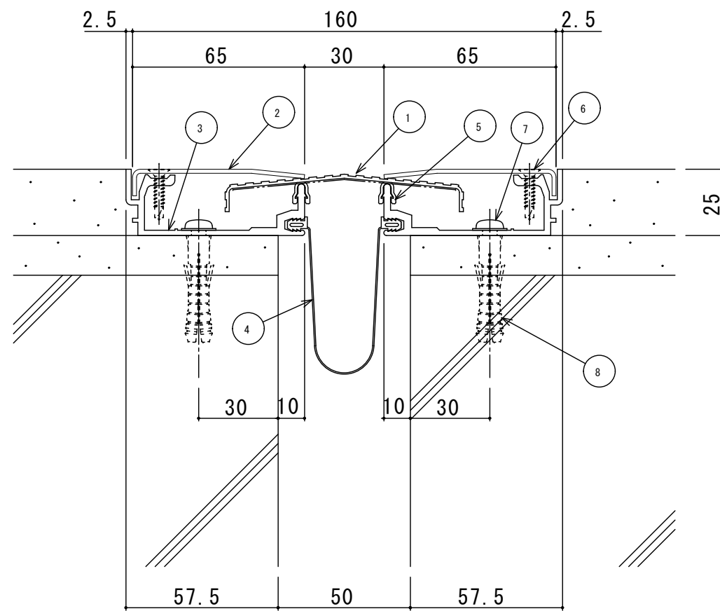
S50-FH 断面図
