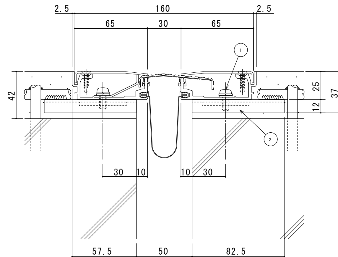
S50-FHA-AS 断面図
