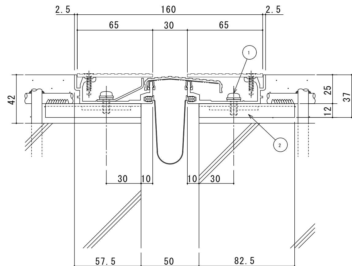
S50-FHJA-AS 断面図
