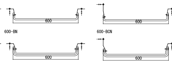
【600mm用 耐火帯】
