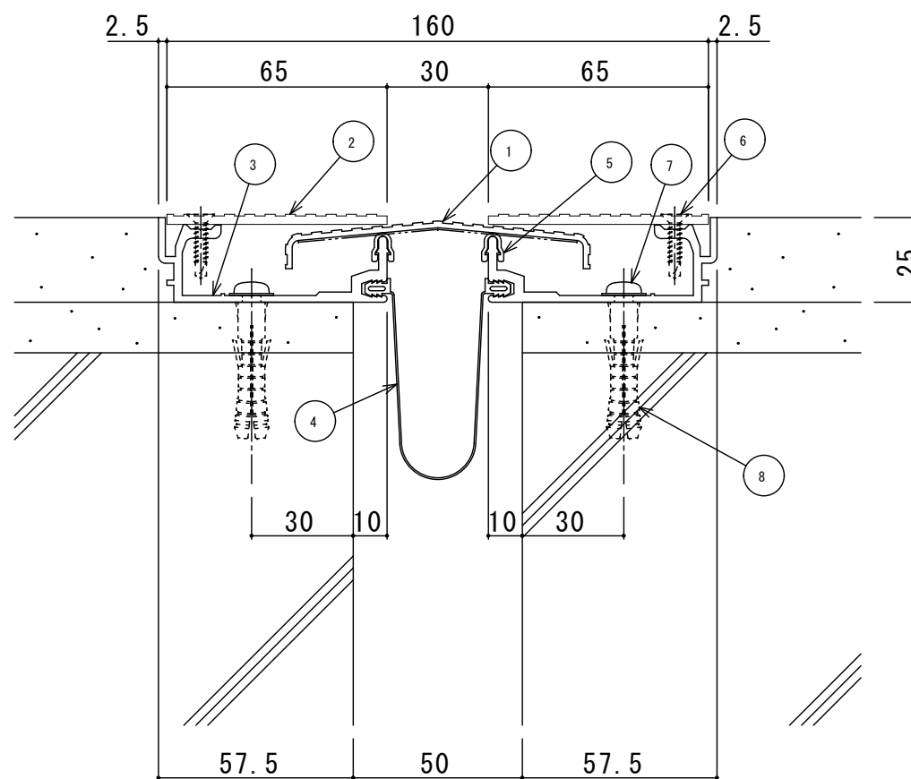
S50-FHJ 断面図
