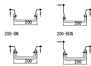
【200mm用 耐火帯】
