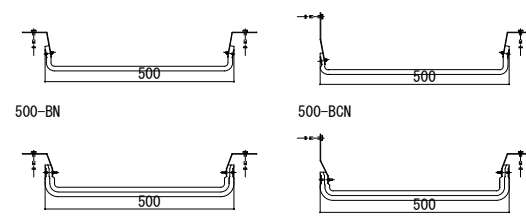
【500mm用 耐火帯】
