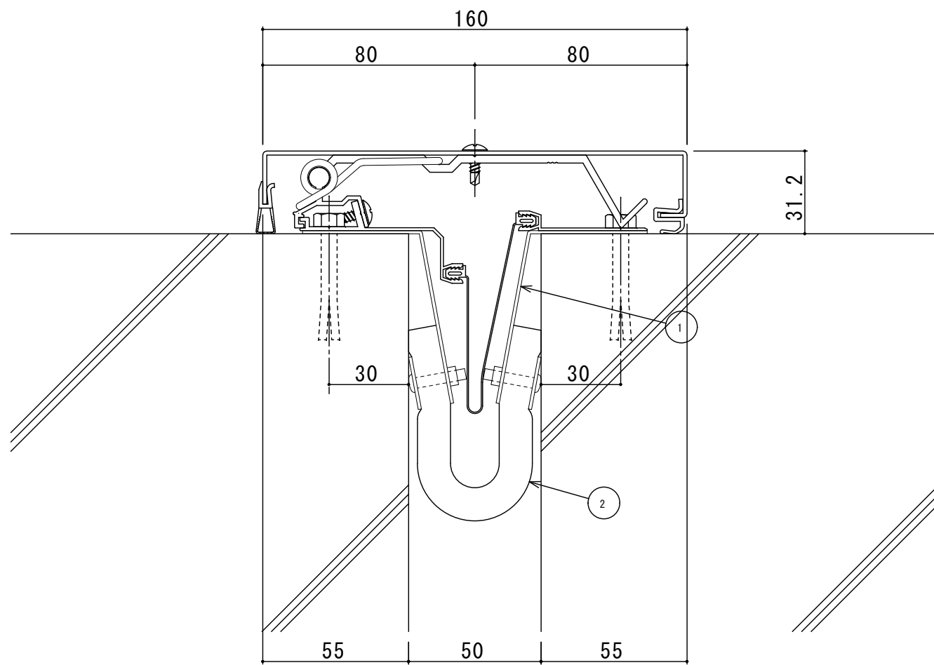
S50-EH（遮炎仕様） 断面図
