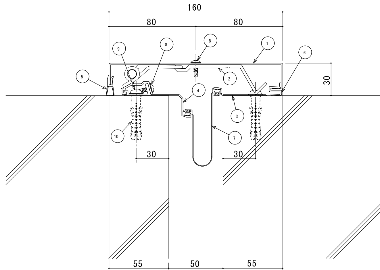
S50-EH 断面図
