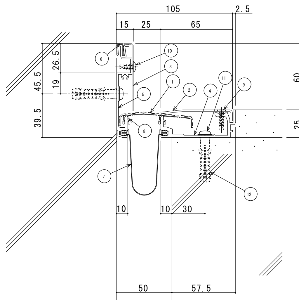
S50-FCH 断面図
