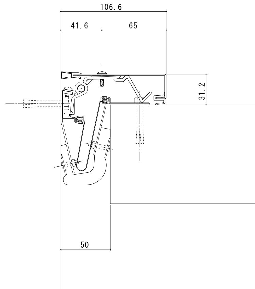
S50-ECH（特殊形状金具遮炎仕様）
