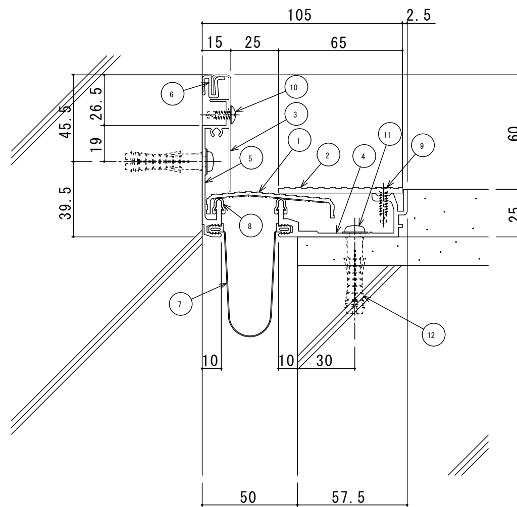
S50-FCHJ 断面図
