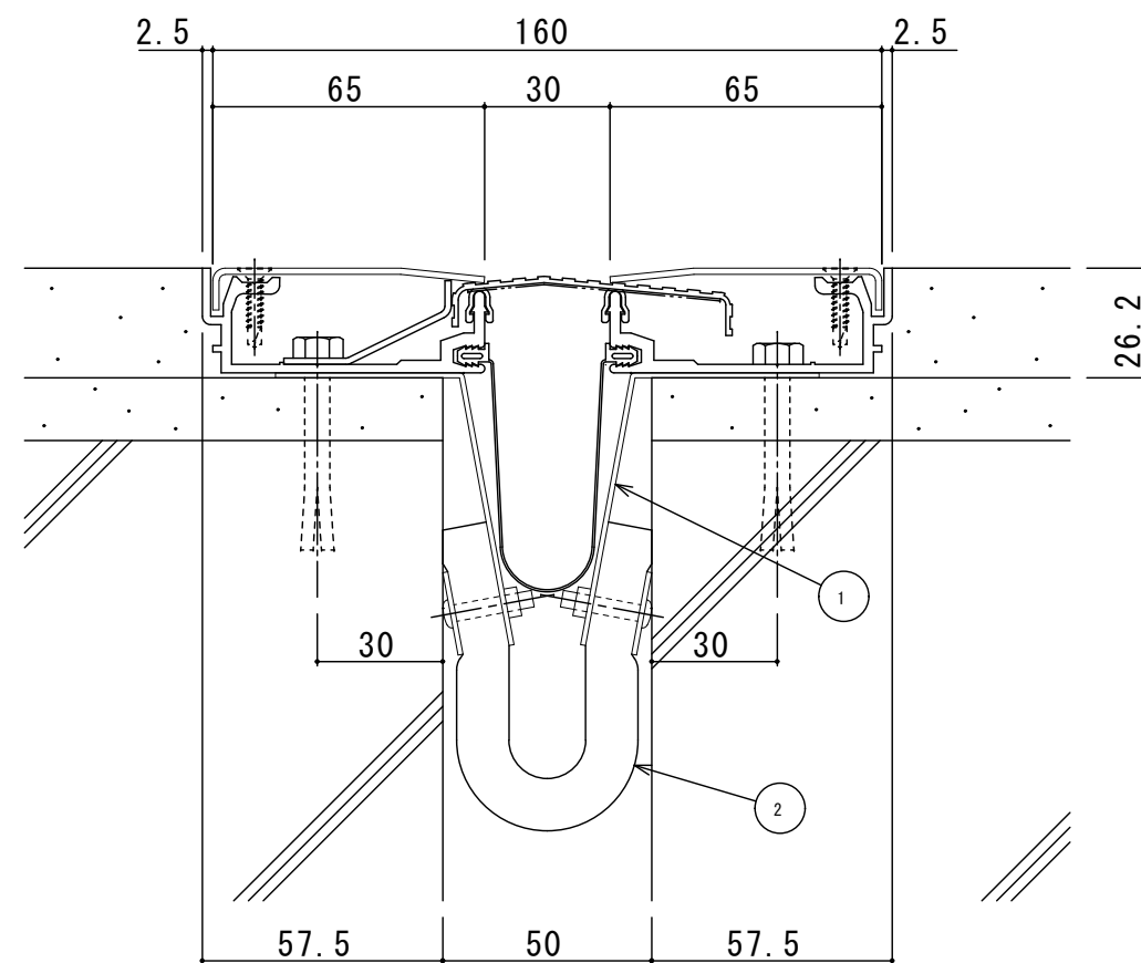
S50-FH-AS（遮炎仕様） 断面図
