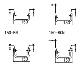
【150mm用 耐火帯】
