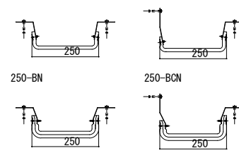
【250mm用 耐火帯】
