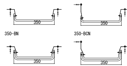
【350mm用 耐火帯】
