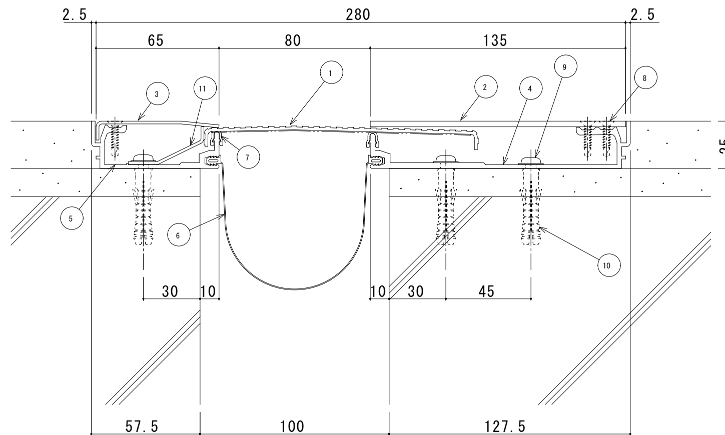
S100-FH-AS 断面図
