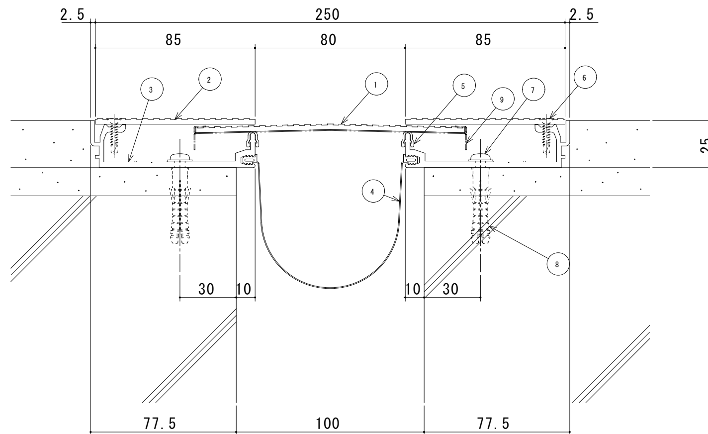
S100-FHJ 断面図
