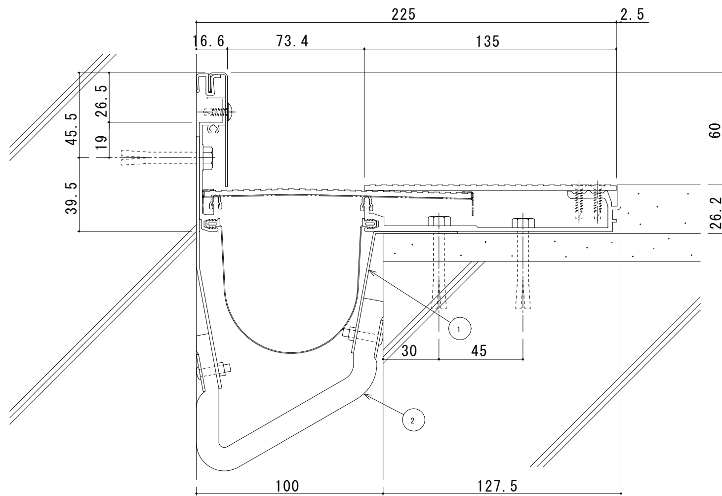
S100-FCHJ(遮炎仕様) 断面図
