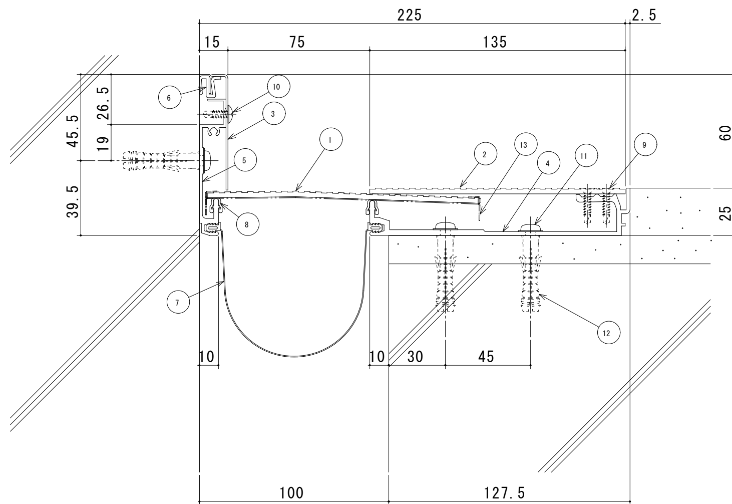
S100-FCHJ 断面図
