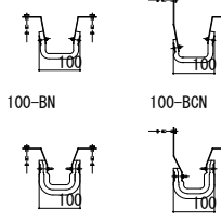
【100mm用 耐火帯】
