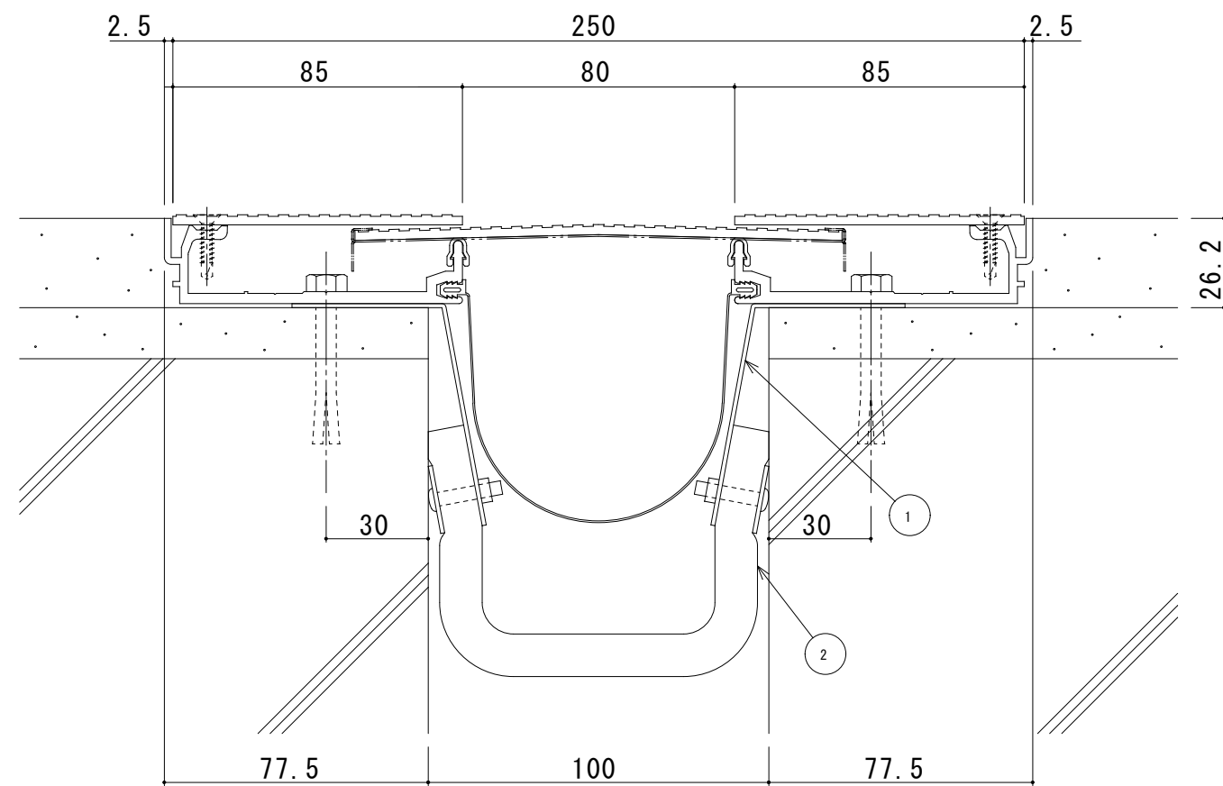
S100-FHJ(遮炎仕様) 断面図
