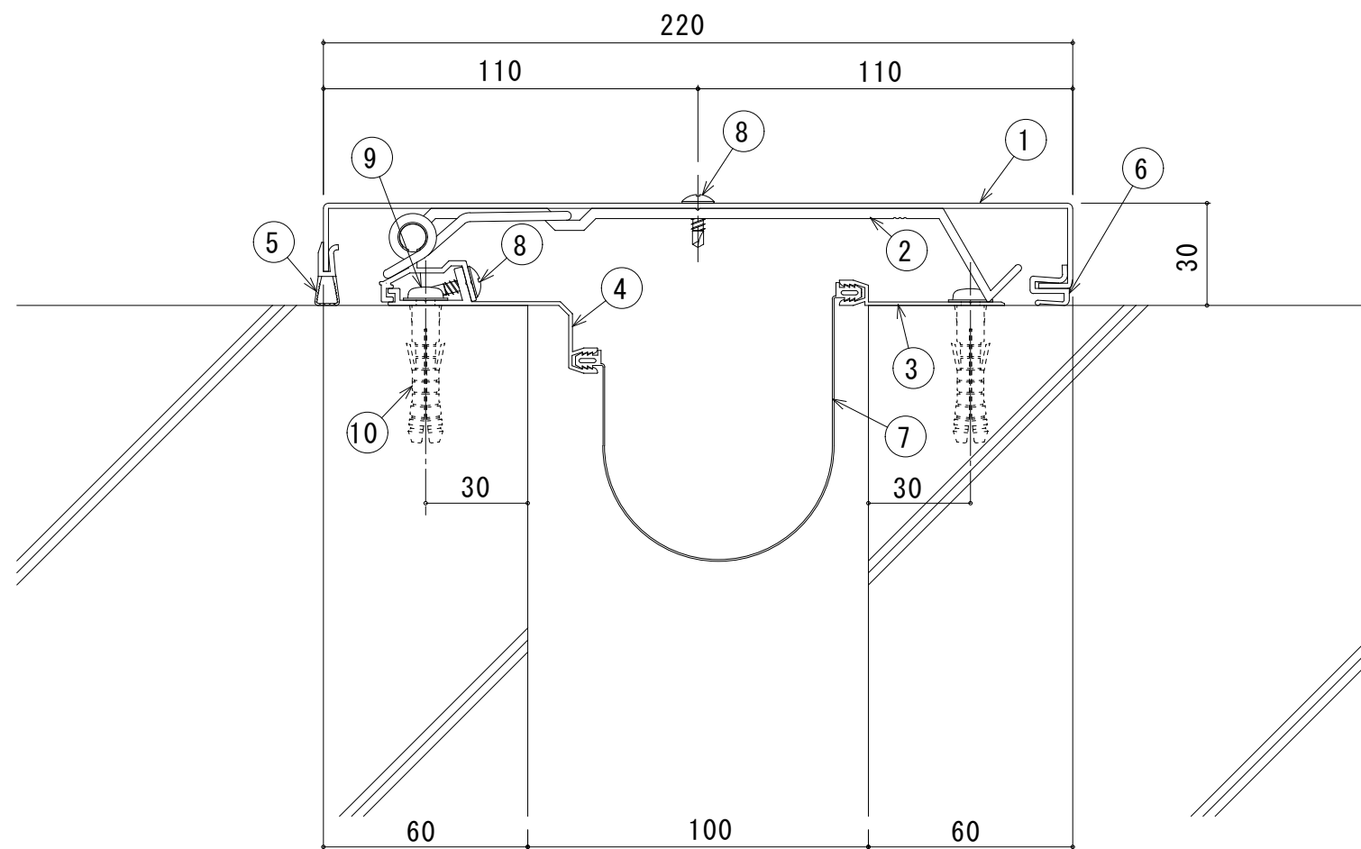
S100-EH 断面図
