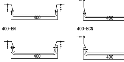
【400mm用 耐火帯】
