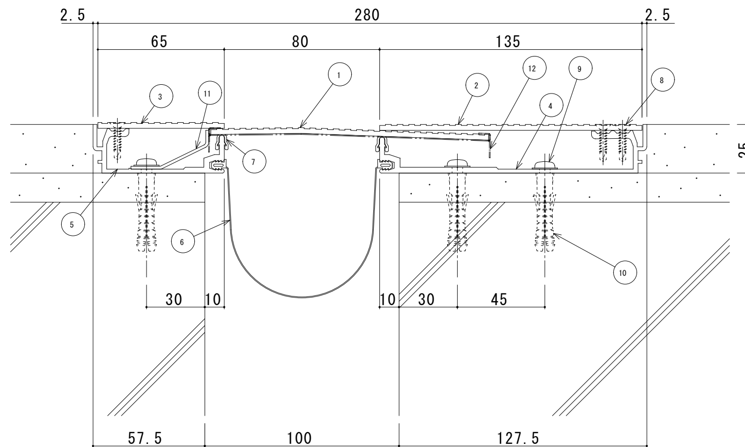
S100-FHJ-AS 断面図
