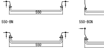
【550mm用 耐火帯】
