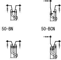
【50mm用 耐火帯】
