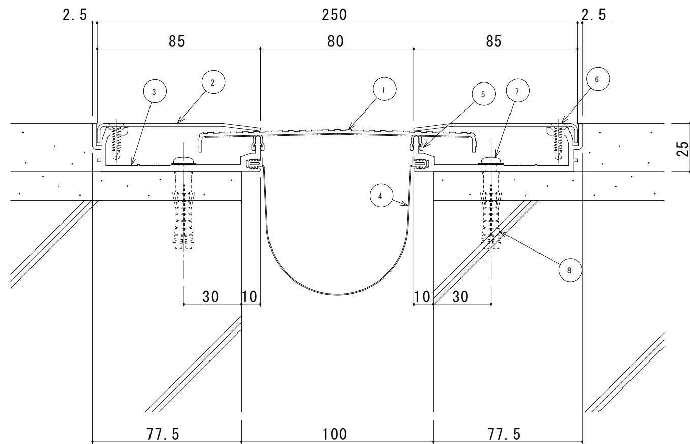
S100-FH 断面図
