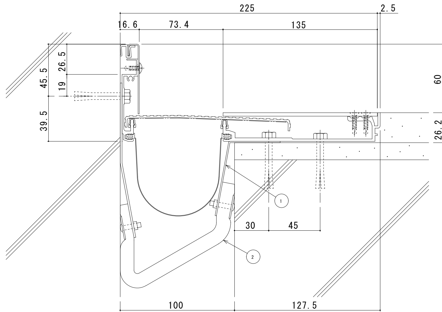
S100-FCH(遮炎仕様) 断面図
