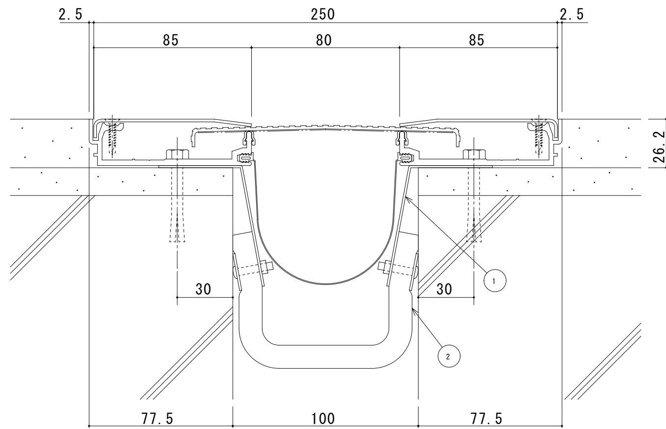
S100-FH(遮炎仕様) 断面図
