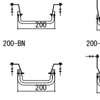
【200mm用 耐火帯】
