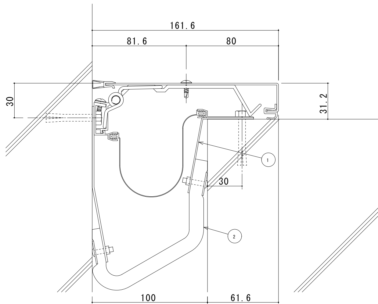
S100-ECH（遮炎仕様） 断面図
