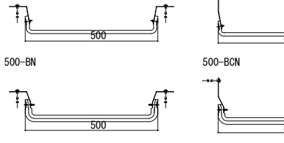
【500mm用 耐火帯】
