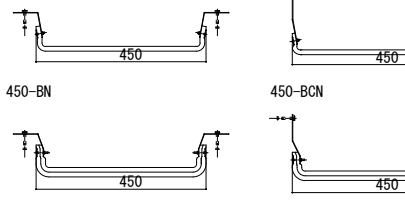
【450mm用 耐火帯】
