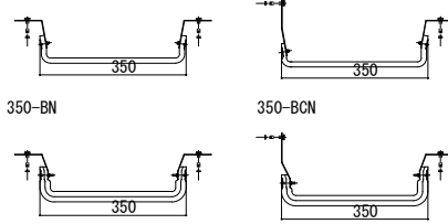
【350mm用 耐火帯】
