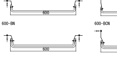
【600mm用 耐火帯】
