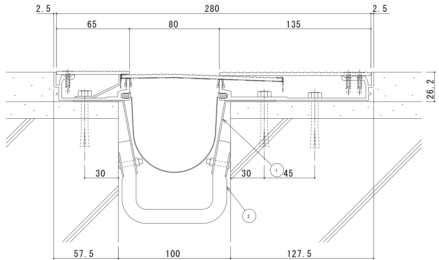
S100-FHJ(遮炎仕様) 断面図
