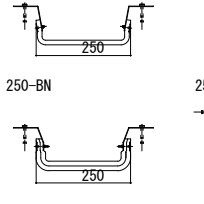
【250mm用 耐火帯】
