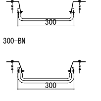
【300mm用 耐火帯】
