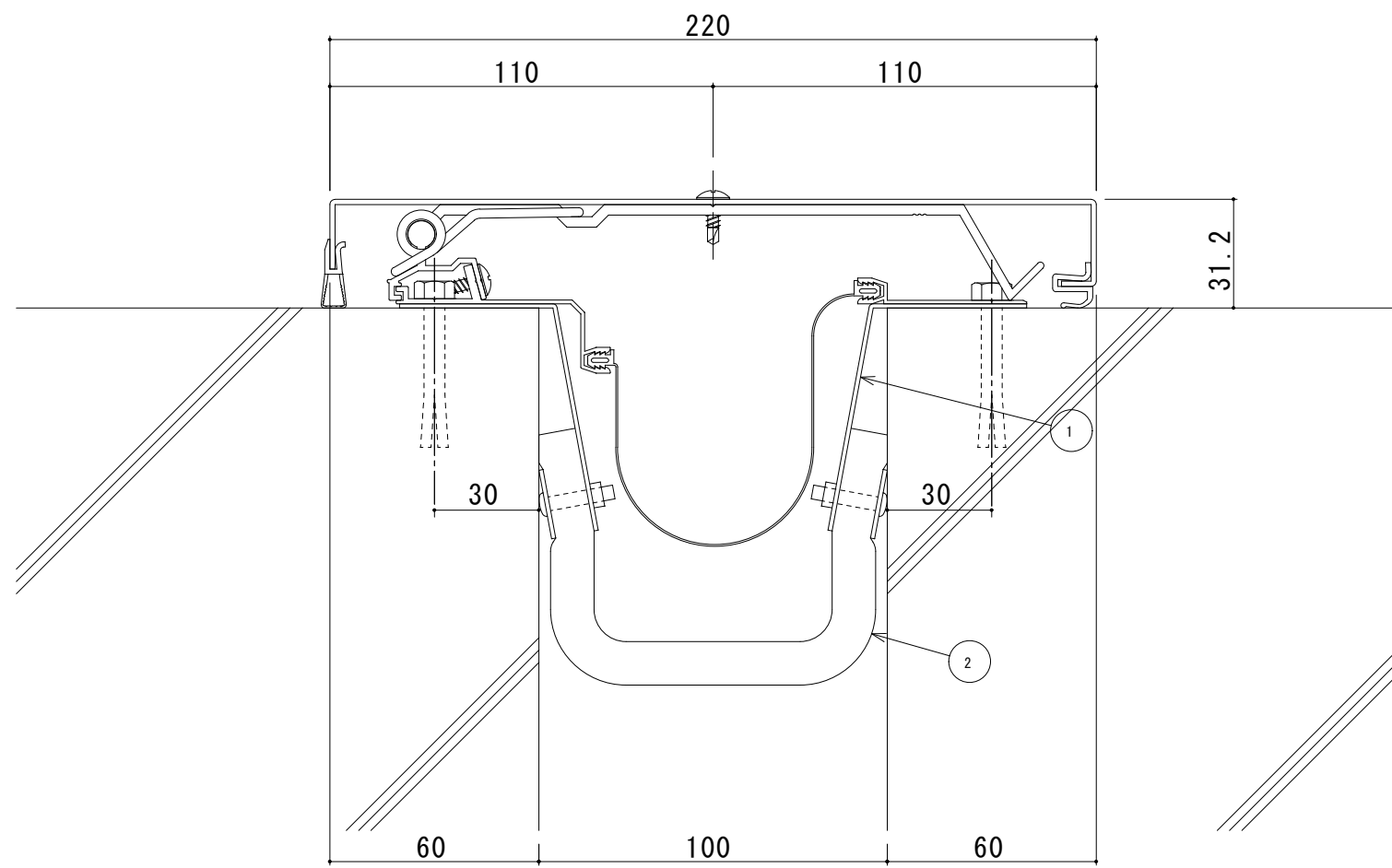
S100-EH（遮炎仕様） 断面図
