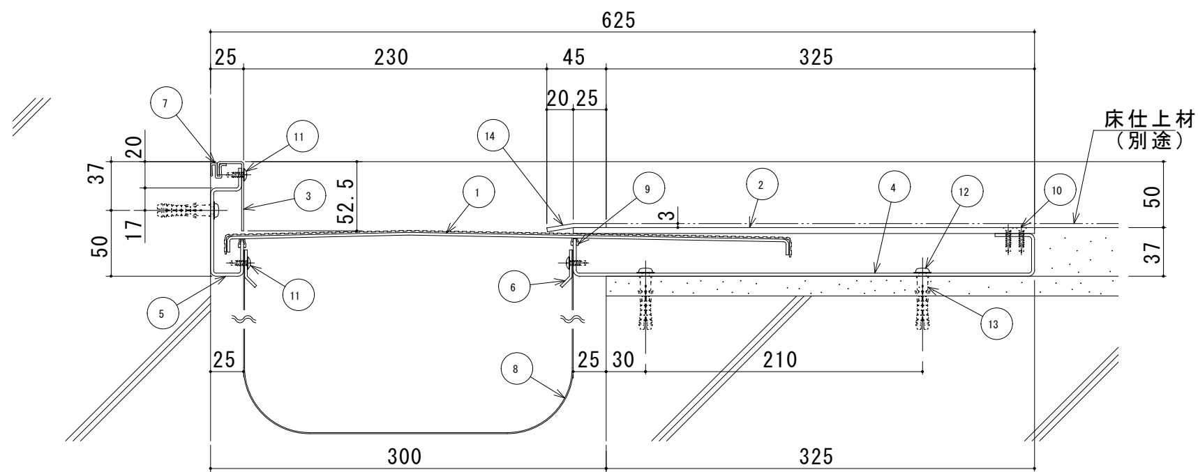
S300-FCHM 断面図
