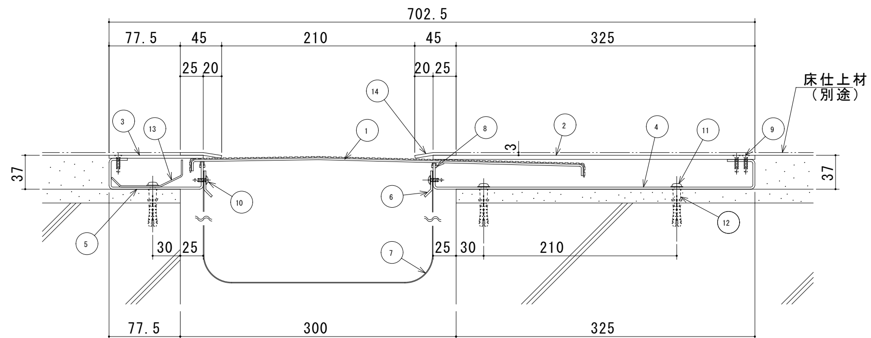
S300-FHM-AS 断面図
