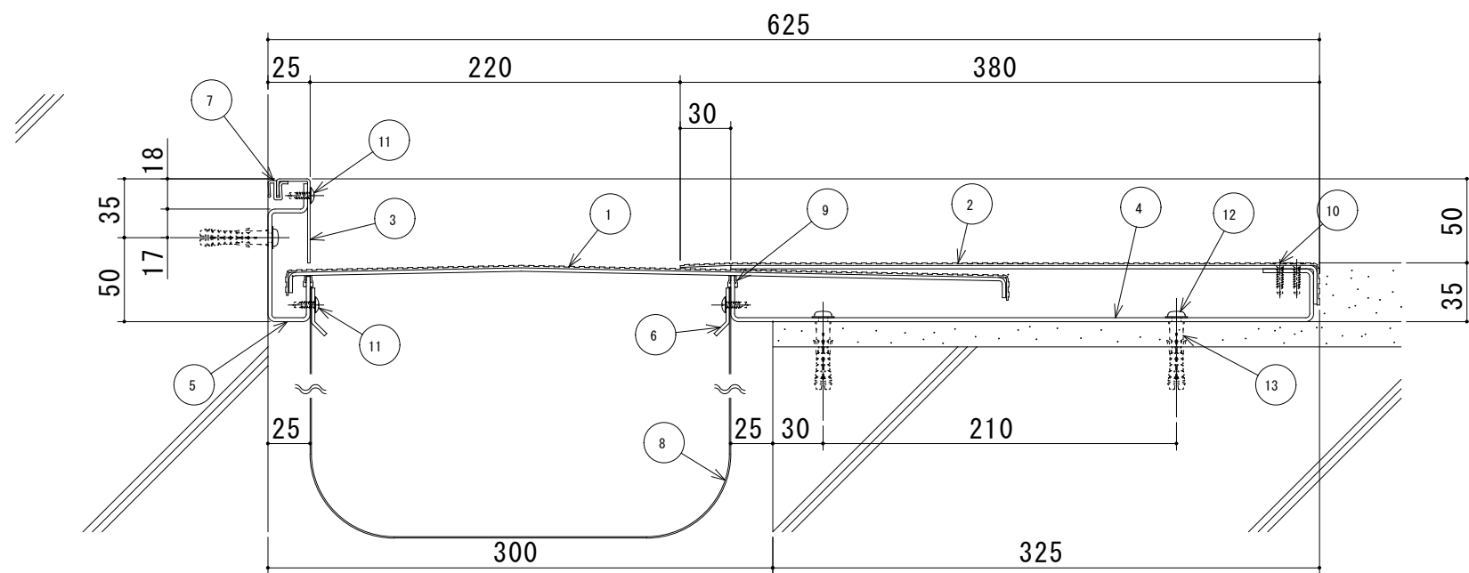
S300-FCH 断面図
