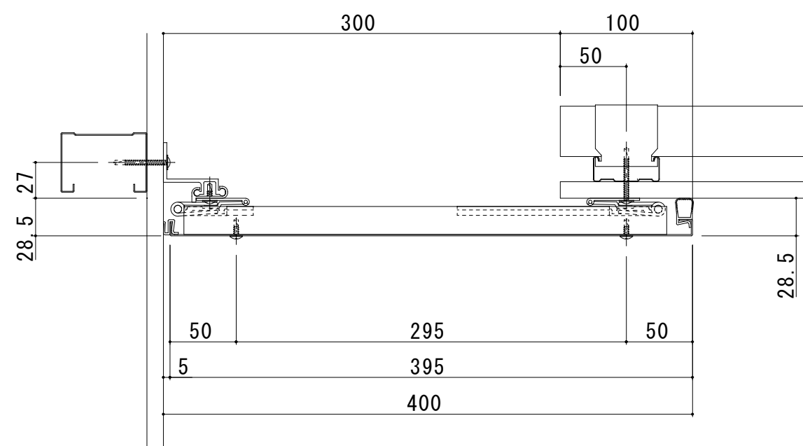
S300-TCE 断面图
