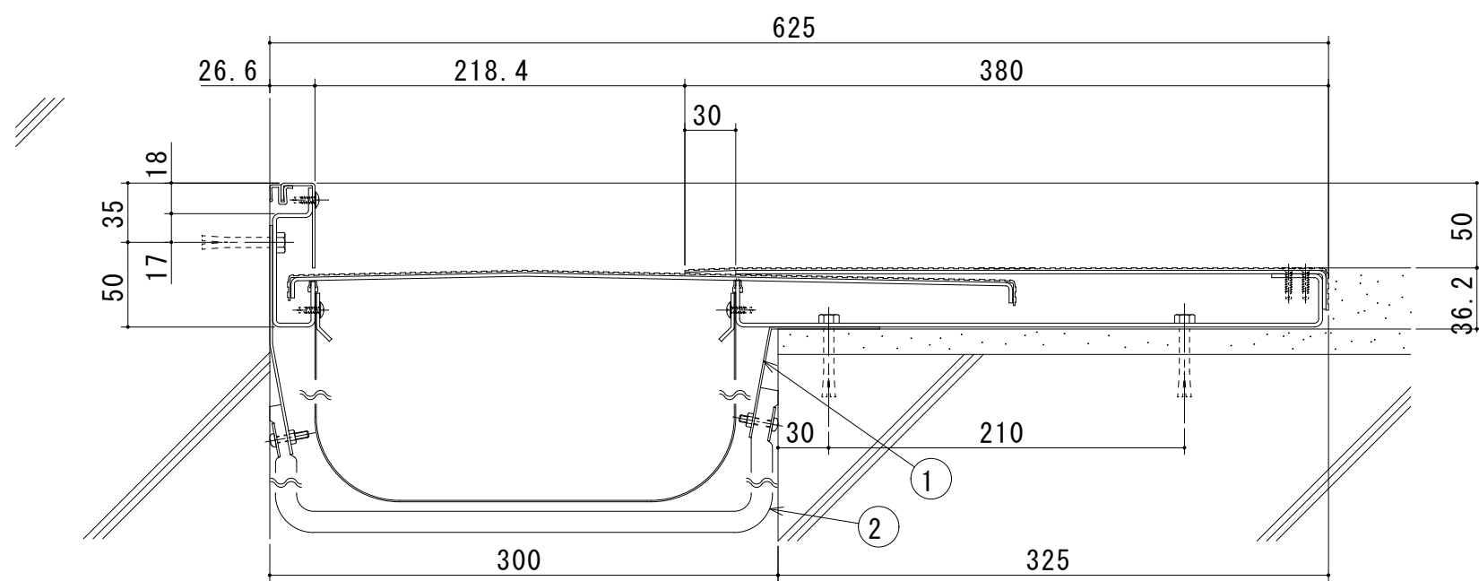
S300-FCH(遮炎仕様) 断面図
