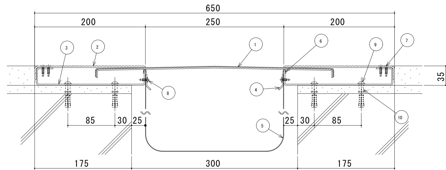
S300-FH 断面図
