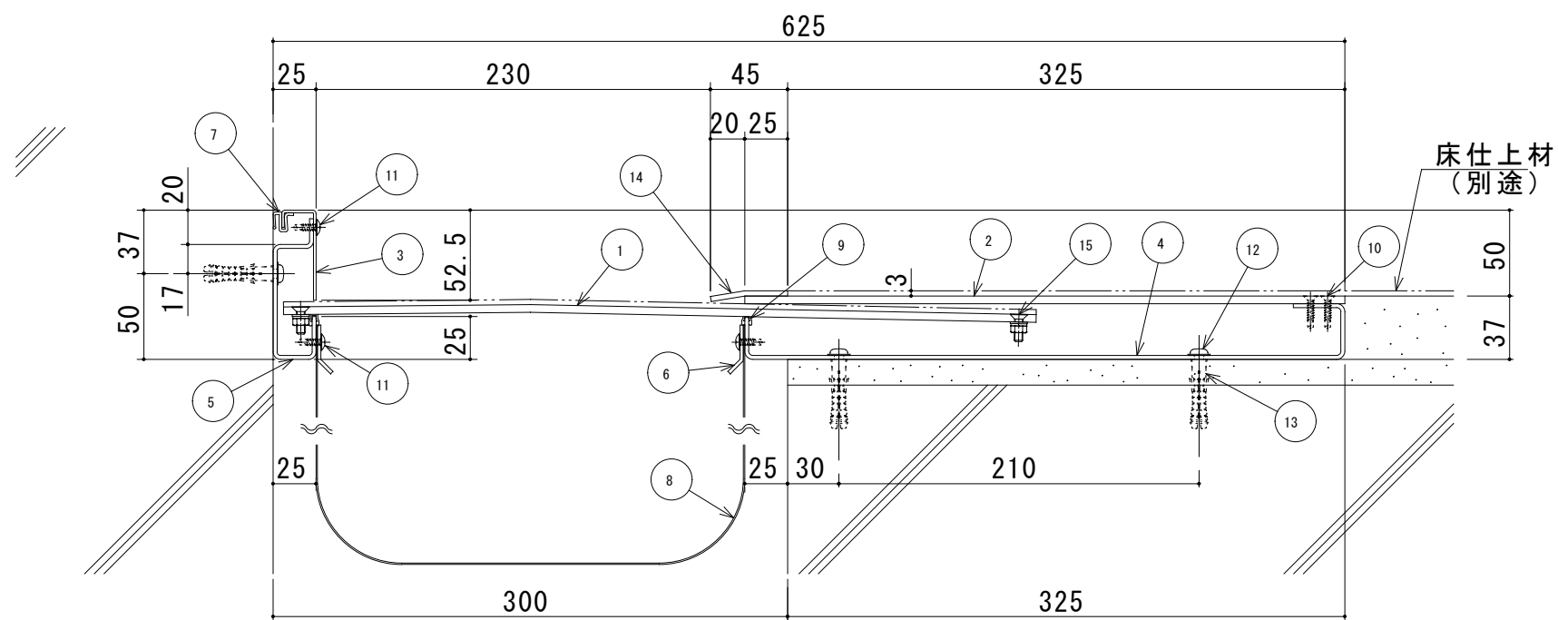
S300-FCHMB 断面図
