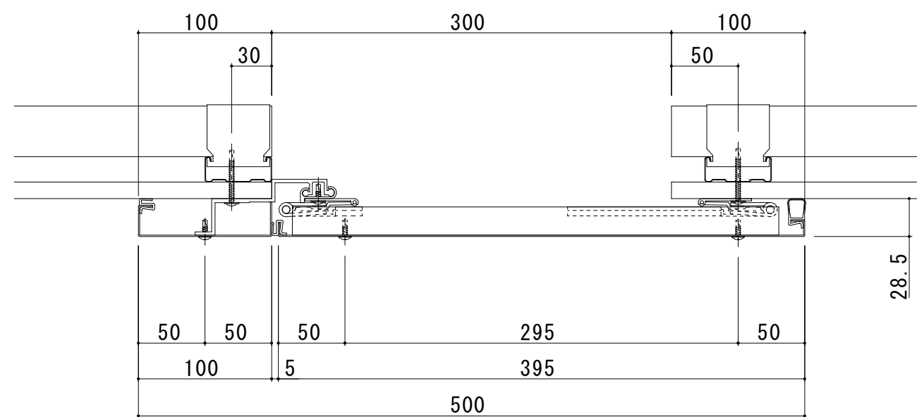
S300-TE 断面图
