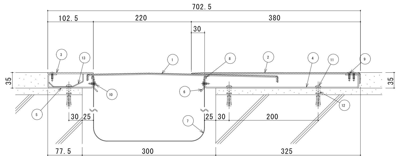
S300-FH-AS 断面図
