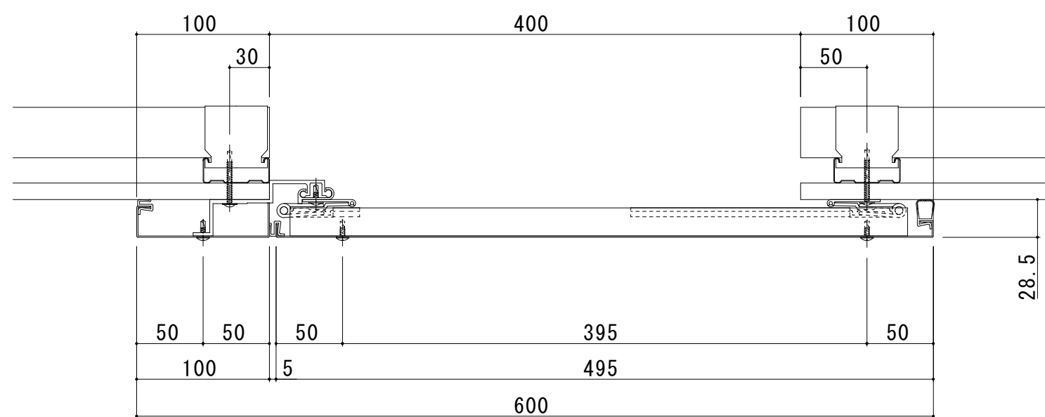
S400-TE 断面图
