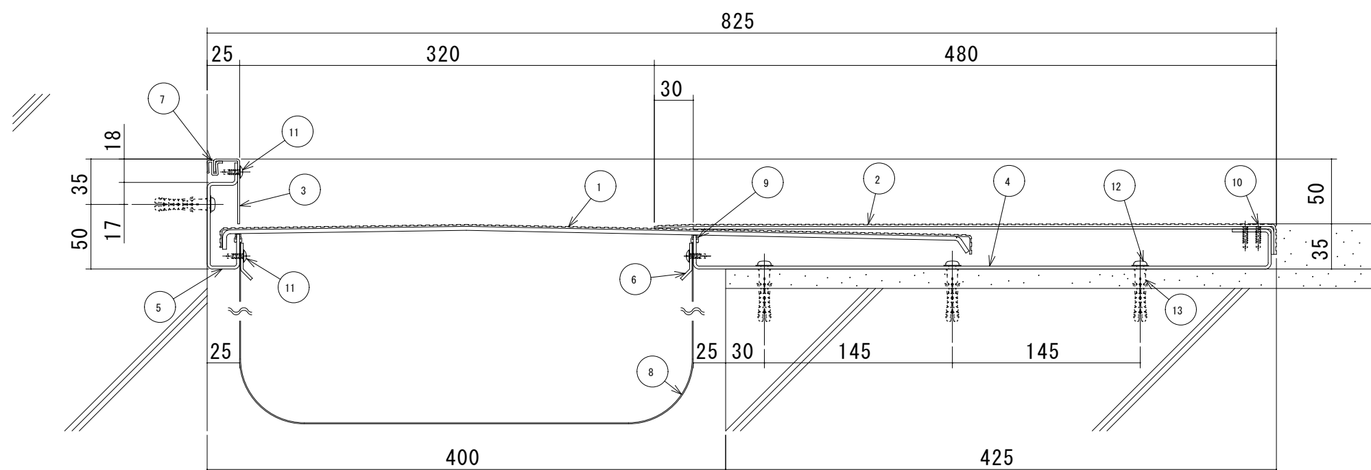
S400-FCH 断面図
