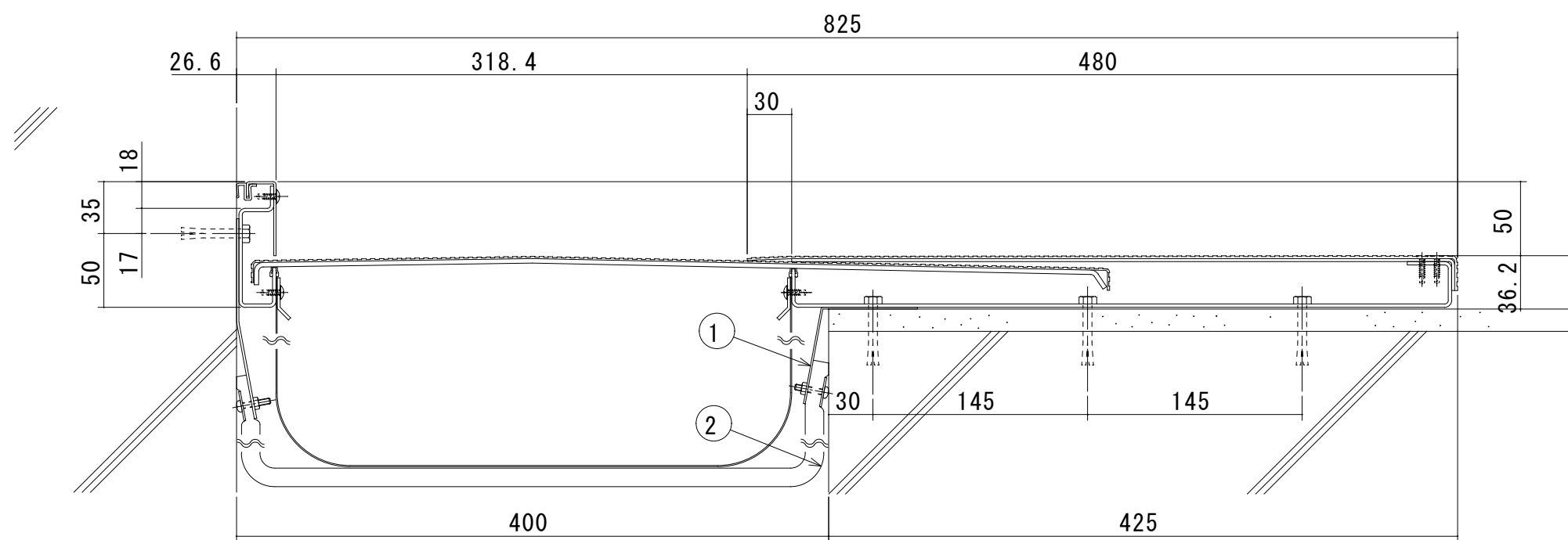
S400-FCH（遮炎仕様） 断面図
