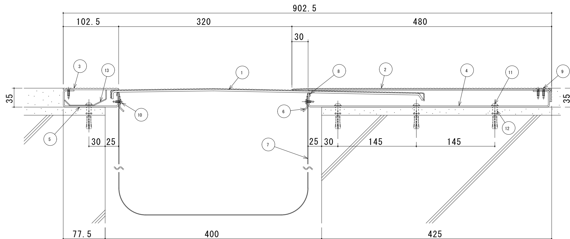
S400-FH-AS 断面図
