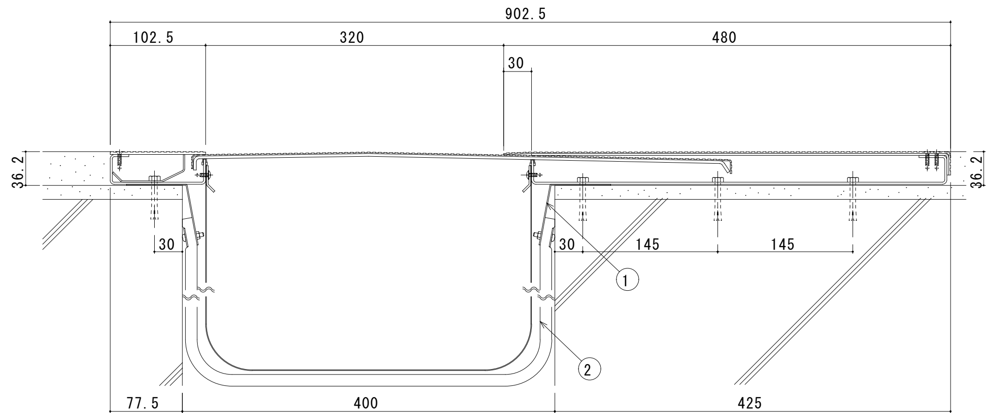
S400-FH-AS（遮炎仕様） 断面図
