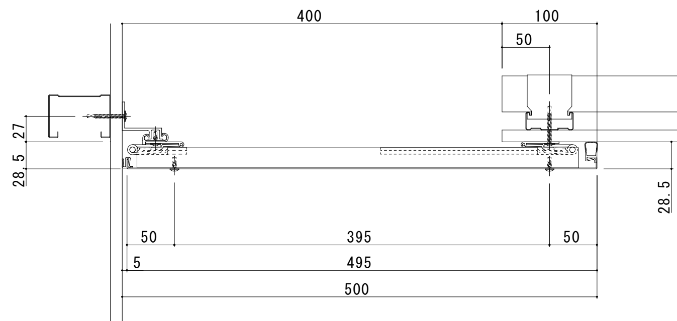
S400-TCE 断面図
