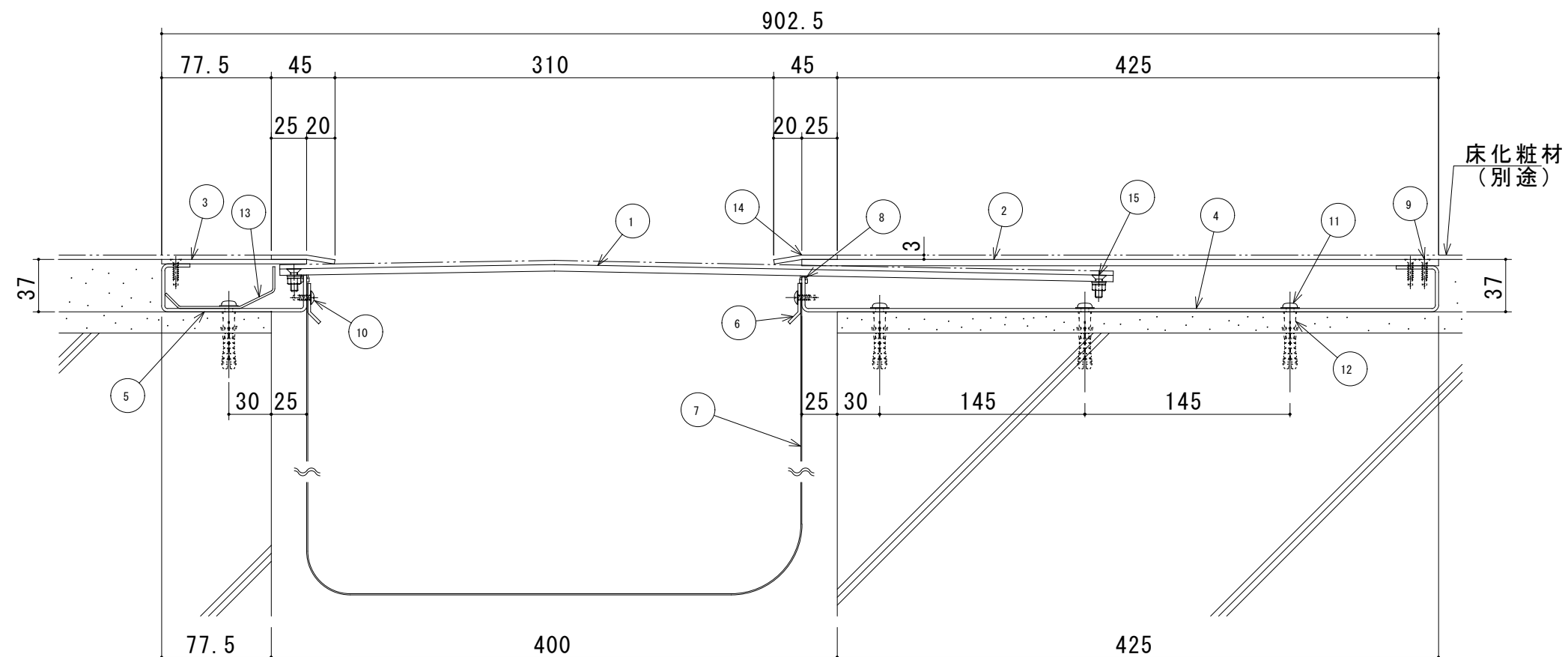
S400-FHMB-AS 断面図
