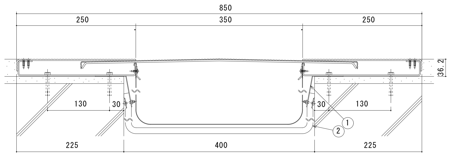
S400-FH（遮炎仕様） 断面図
