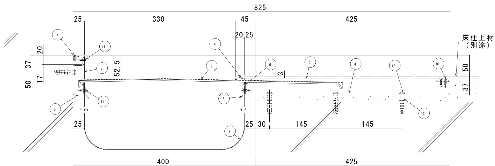
S400-FCHM 断面図
