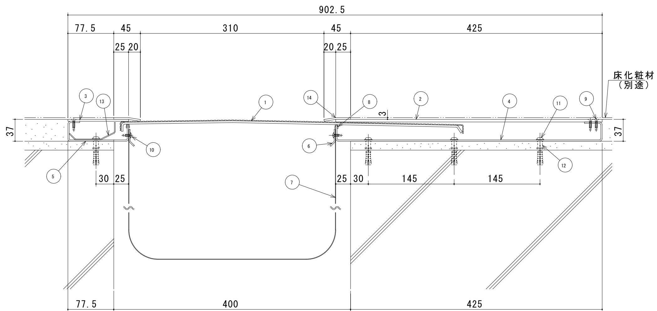
S400-FHM-AS 断面図
