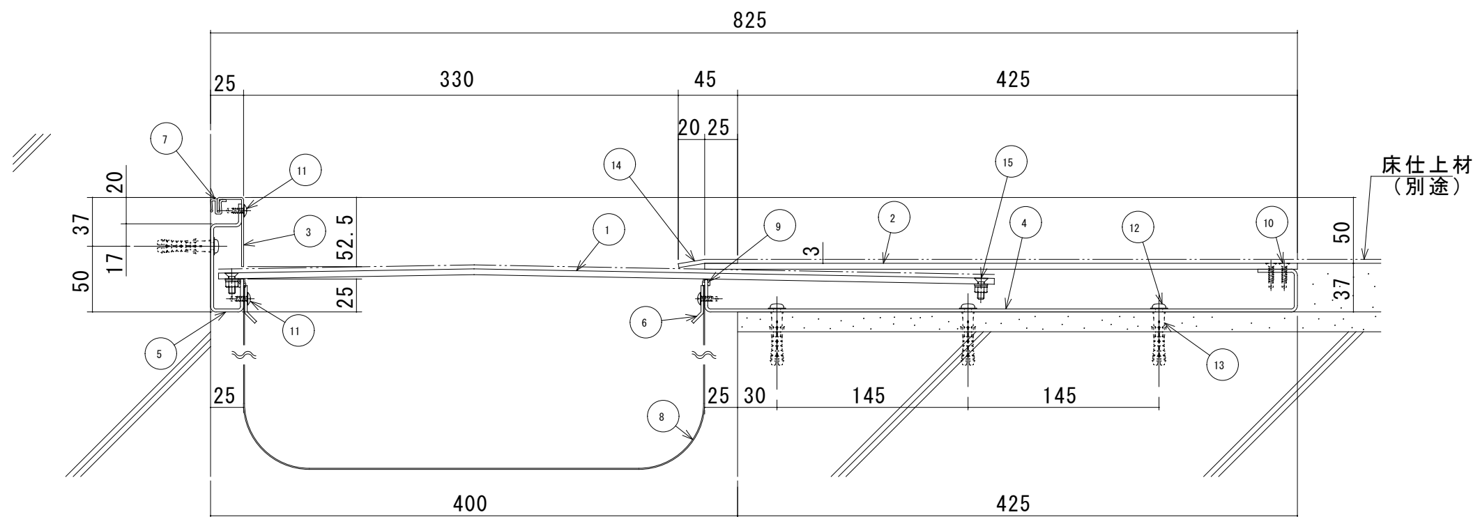
S400-FCHMB 断面図
