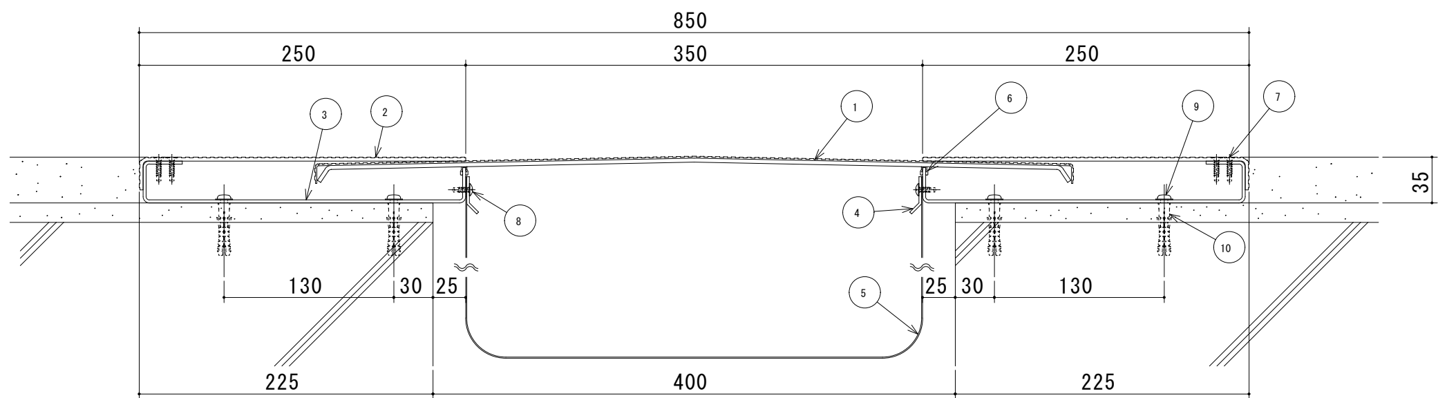
S400-FH 断面図
