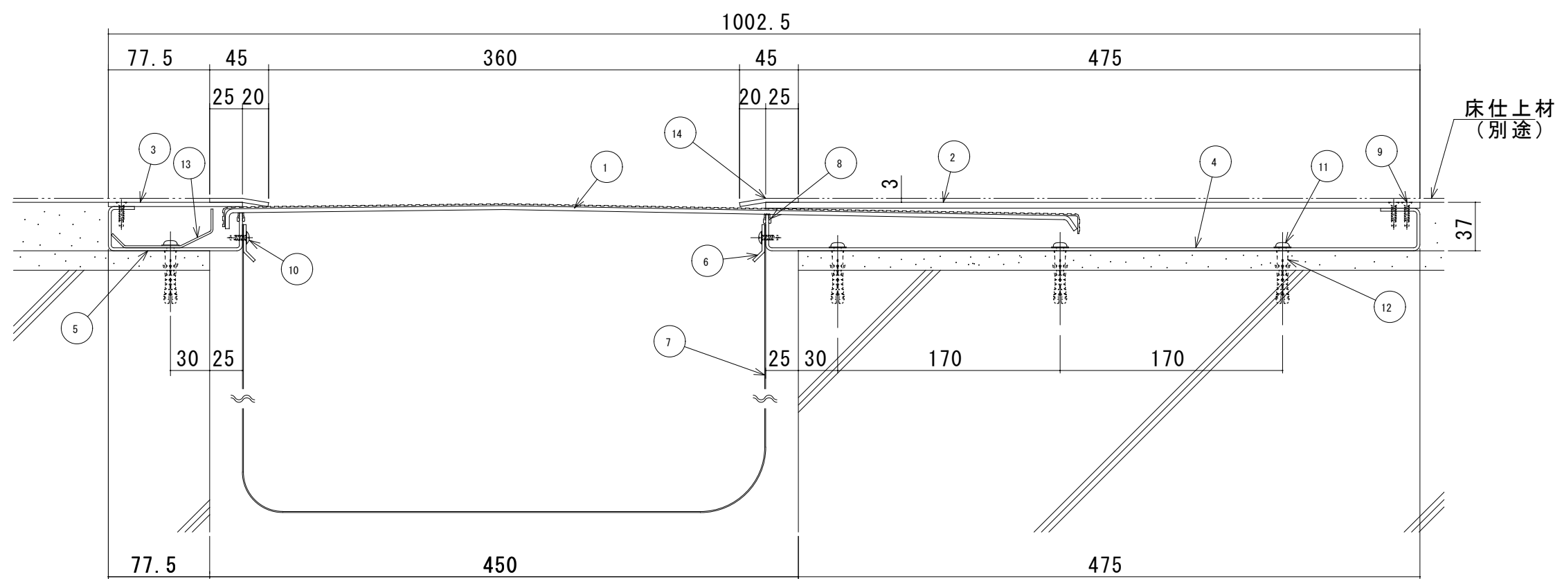
S450-FHM-AS 断面図
