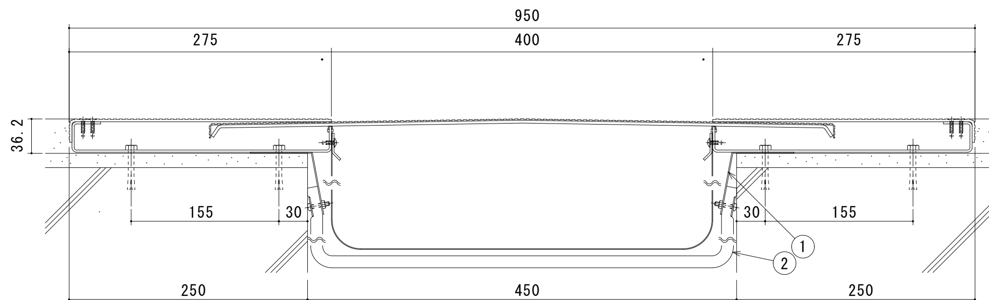
S450-FH（遮炎仕様） 断面図
