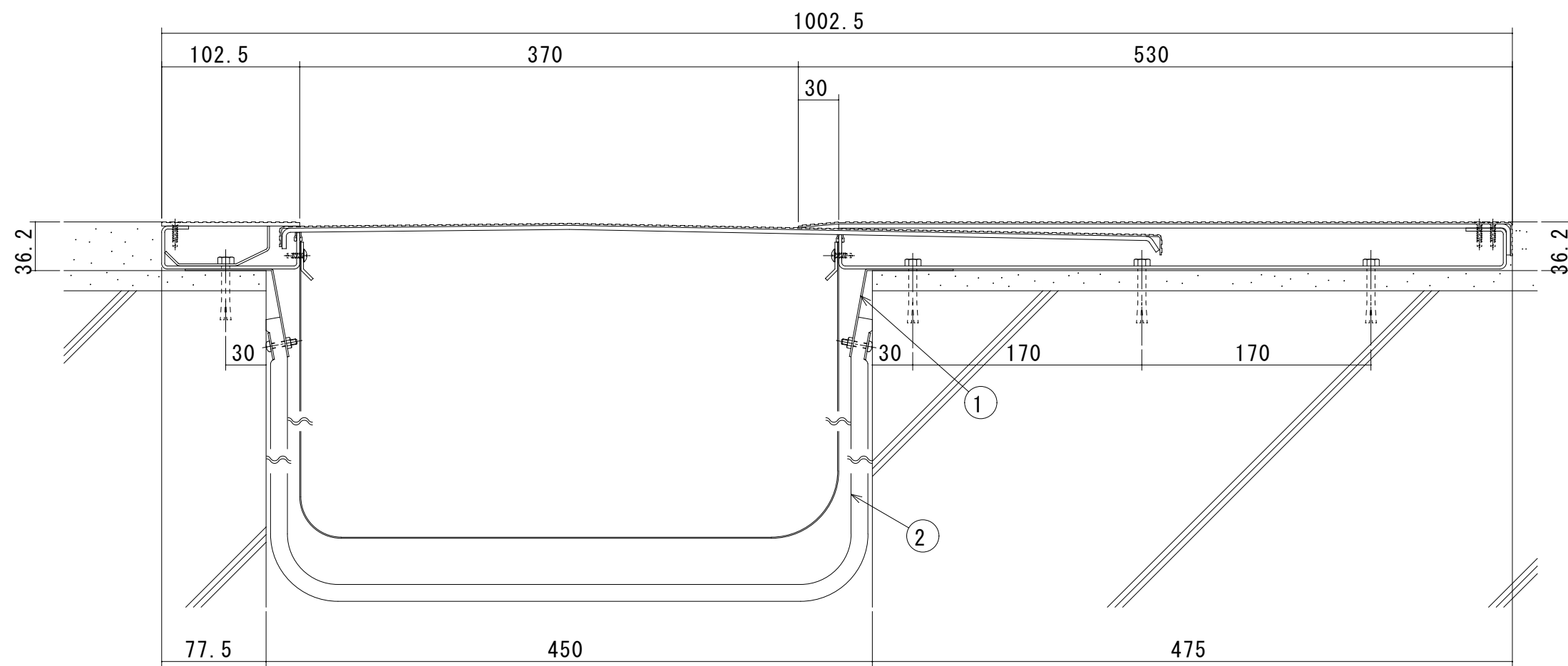
S450-FH-AS (遮炎仕様) 断面図
