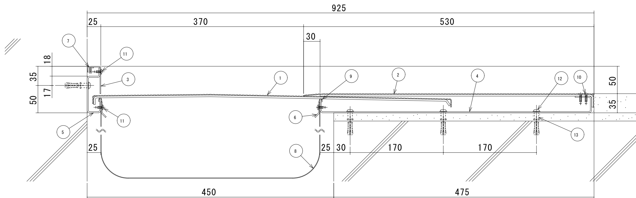
S450-FCH 断面図
