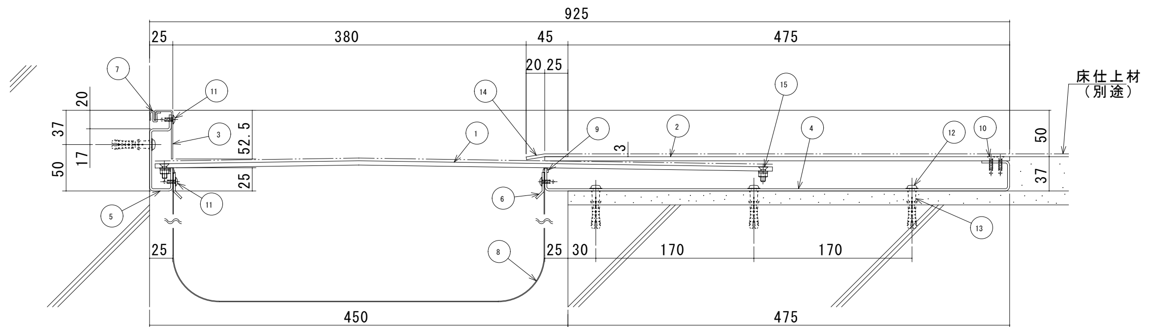
S450-FCHMB 断面図
