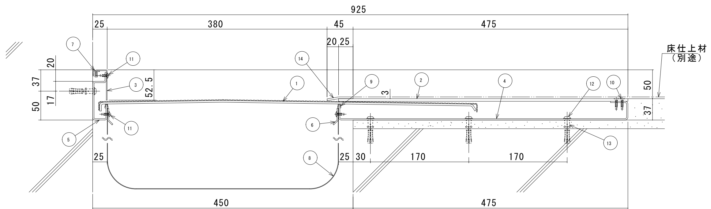
S450-FCHM 断面図
