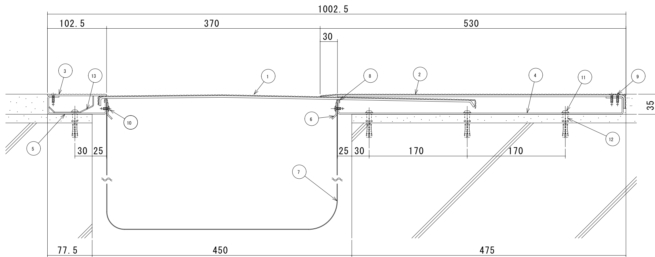
S450-FH-AS 断面図
