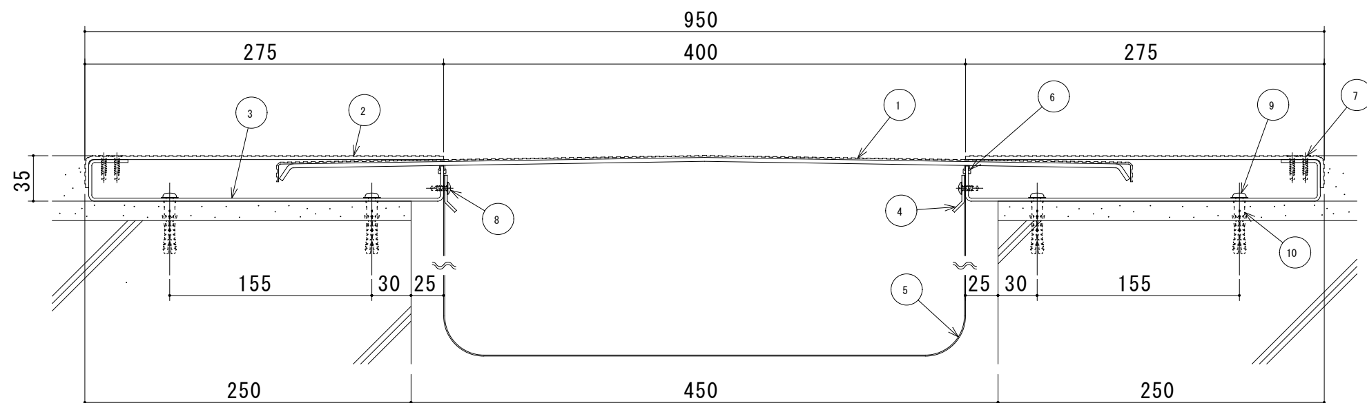
S450-FH 断面図
