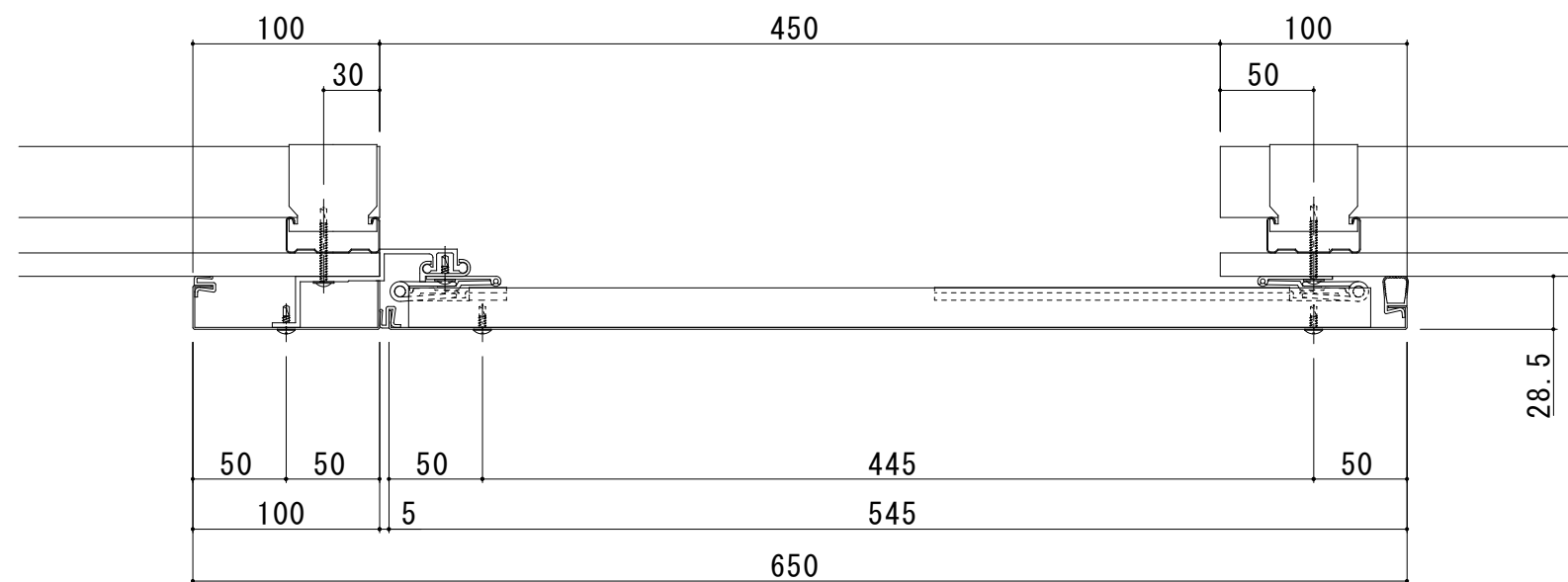
S450-TE 断面图
