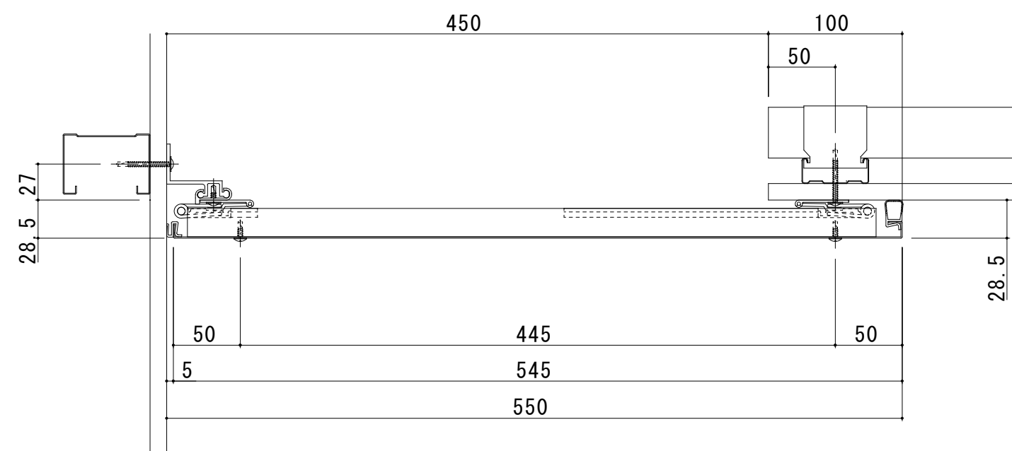
S450-TCE 断面图
