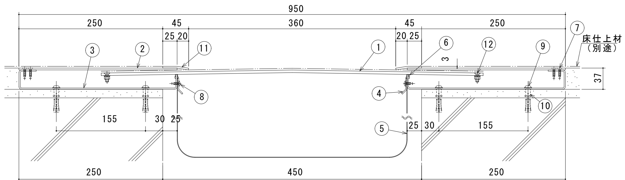
S450-FHMB 断面図
