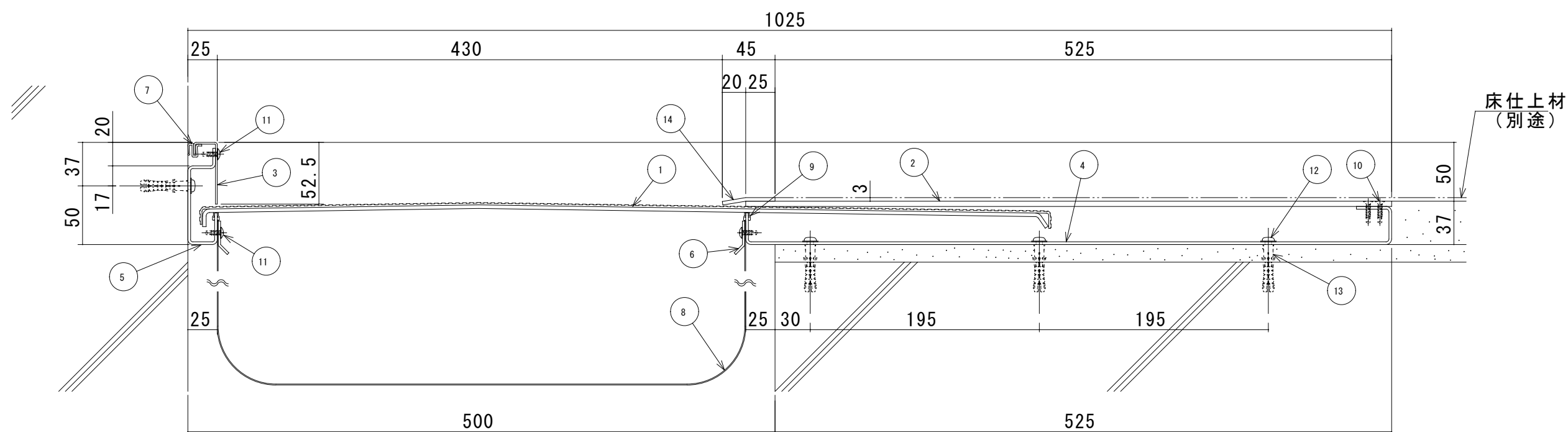
S500-FCHM 断面図
