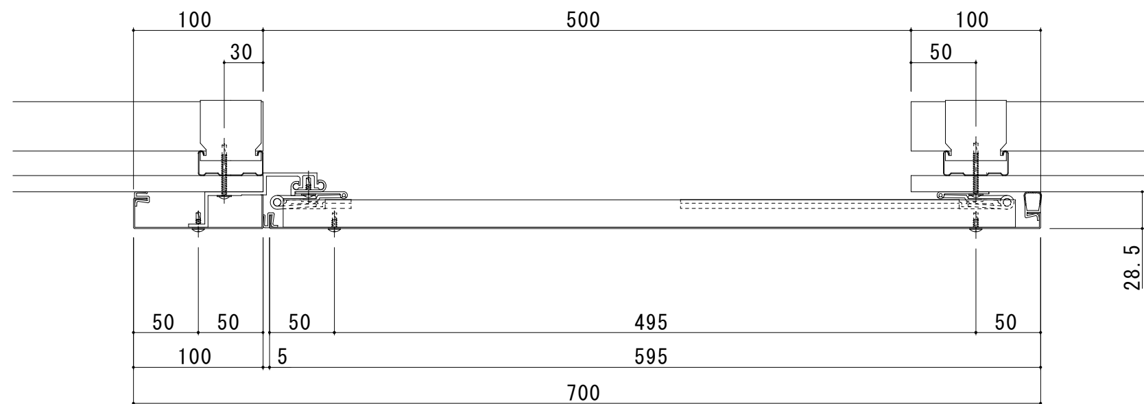
S500-TE 断面图
