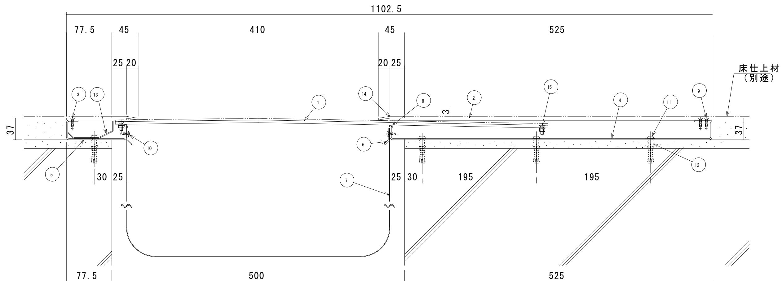
S500-FHMB-AS 断面図
