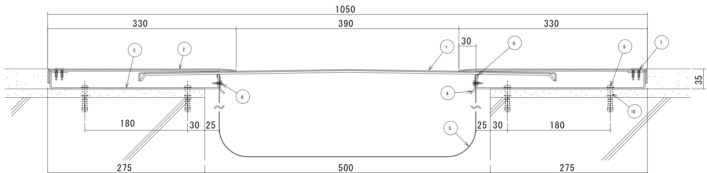
S500-FH 断面図
