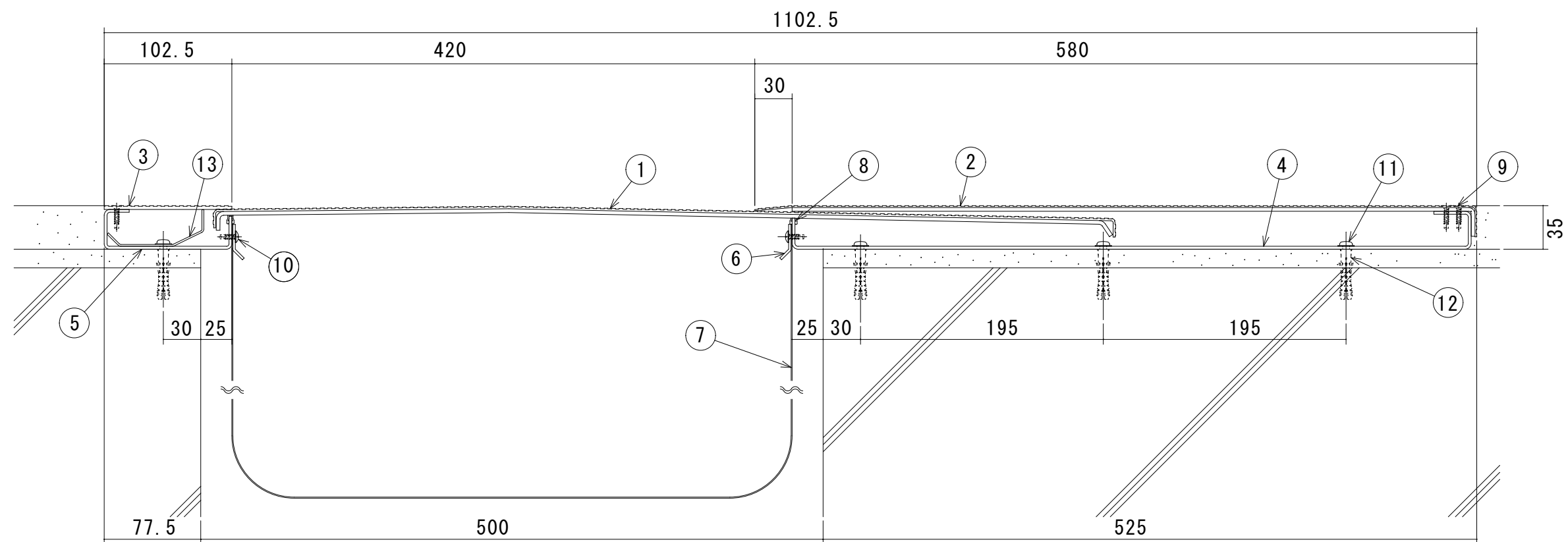
S500-FH-AS 断面図
