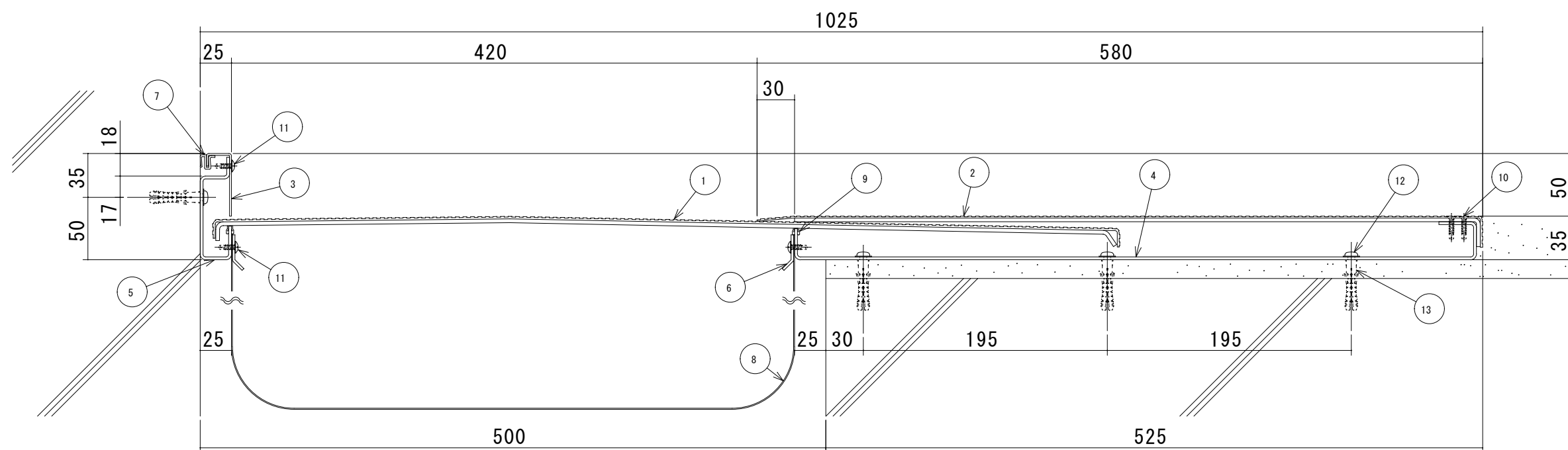
S500-FCH 断面図
