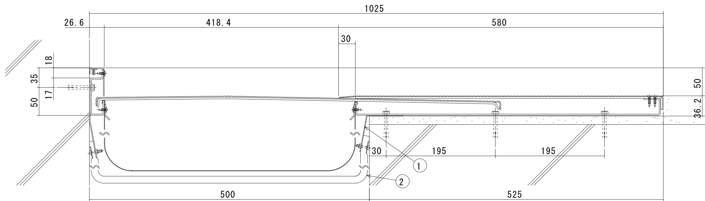
S500-FCH（遮炎仕様） 断面図
