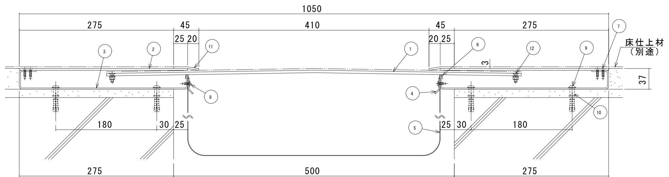
S500-FHMB 断面図
