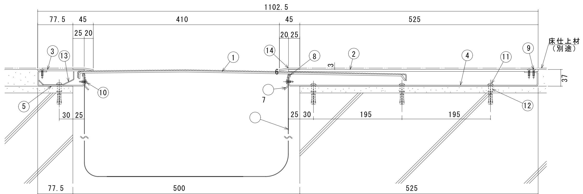
S500-FHM-AS 断面図
