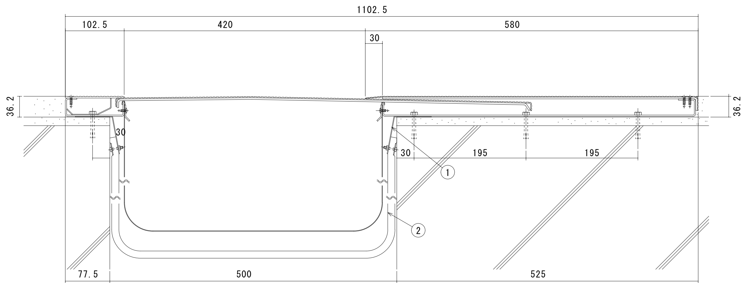
S500-FH-AS（遮炎仕様） 断面図
