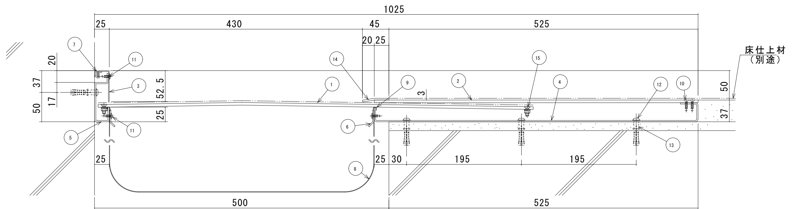
S500-FCHMB 断面図
