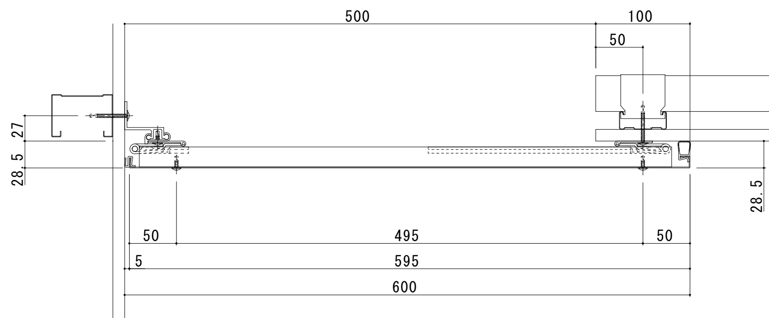
S500-TCE 断面图
