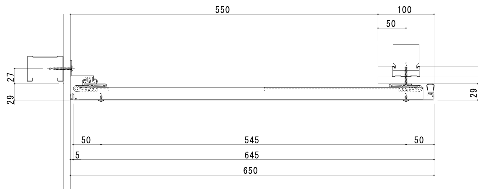
S550-TCE 断面图
