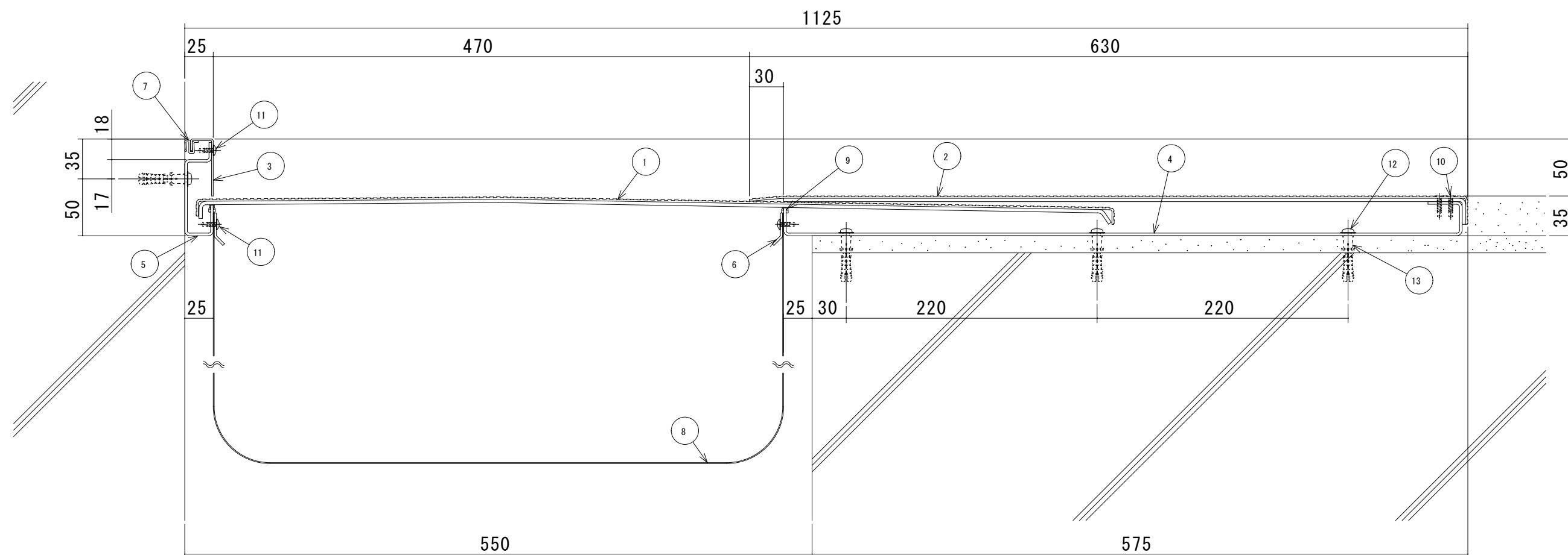
S550-FCH 断面図
