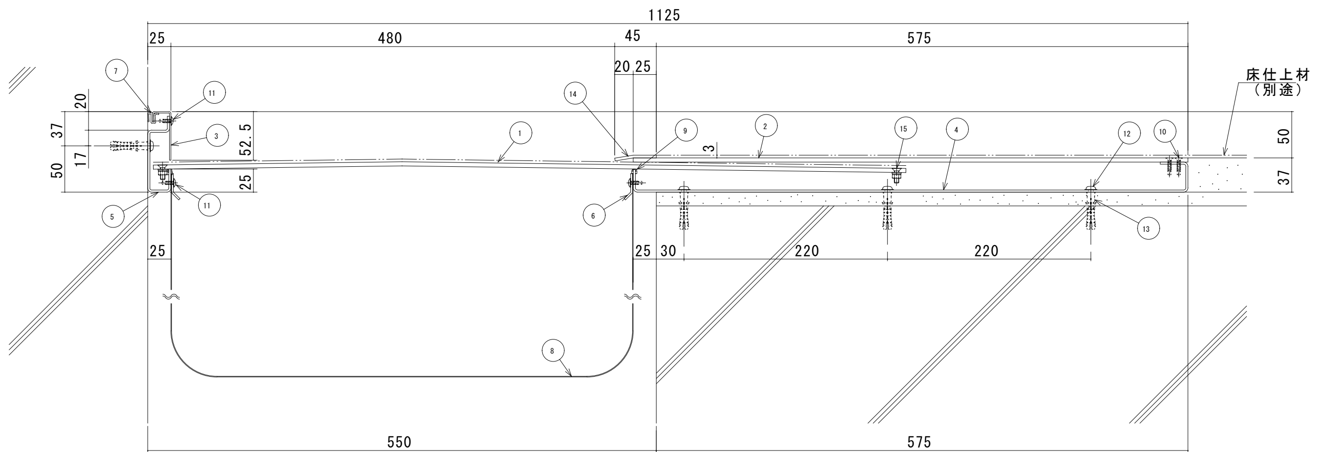
S550-FCHMB 断面図
