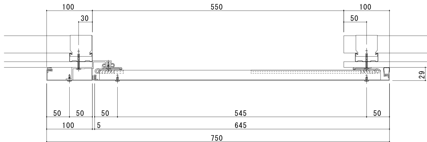
S550-TE 断面图
