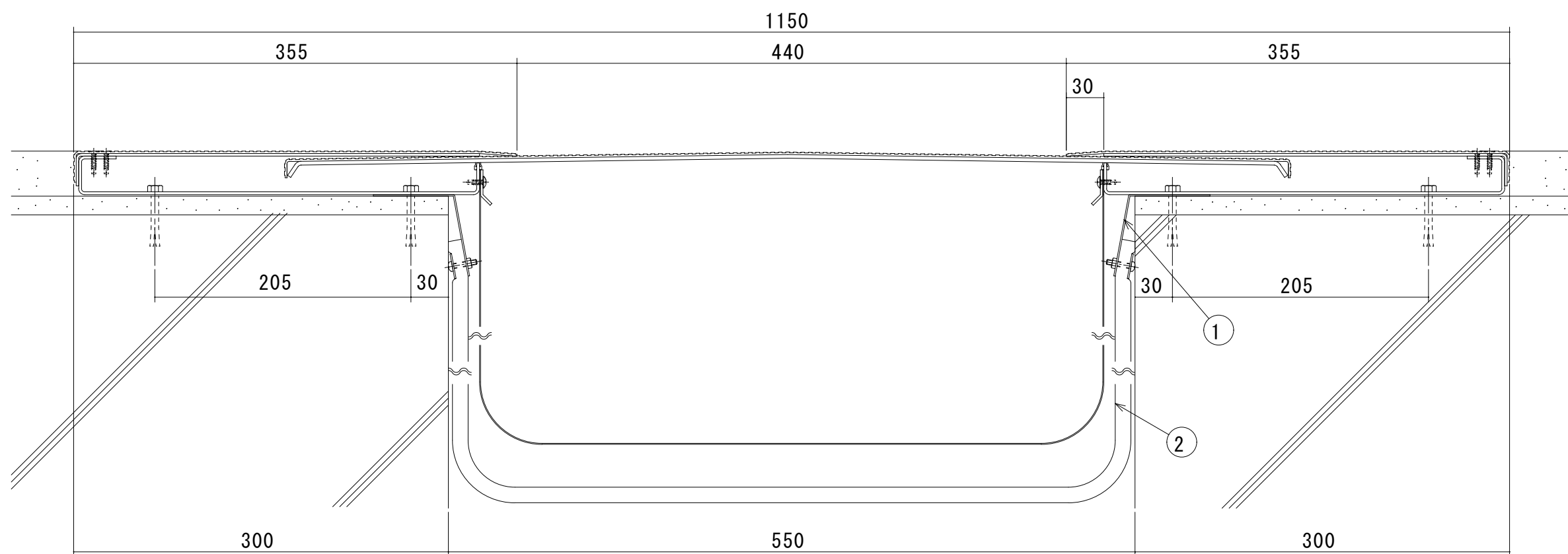
S550-FH（遮炎仕様） 断面図
