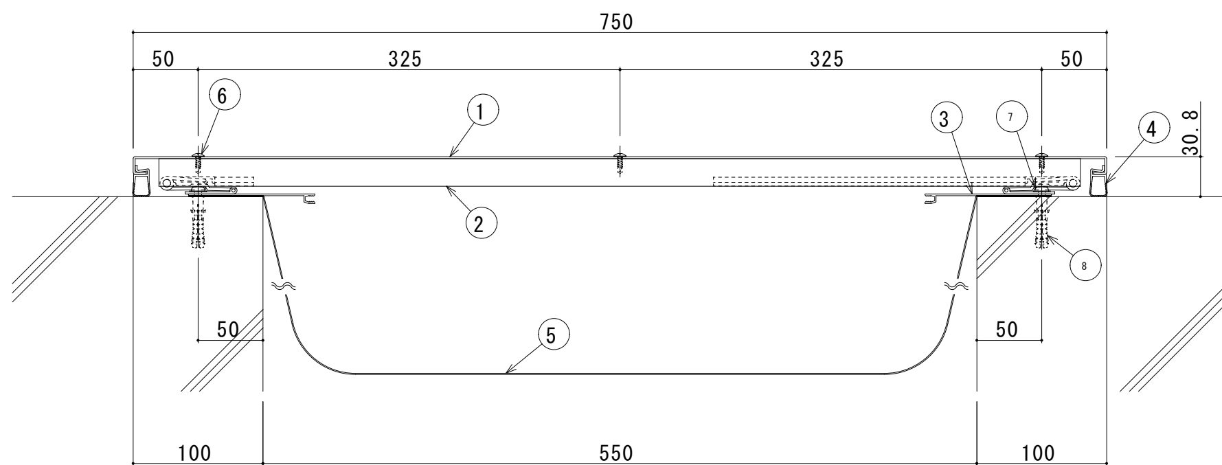
S550-EE 断面図
