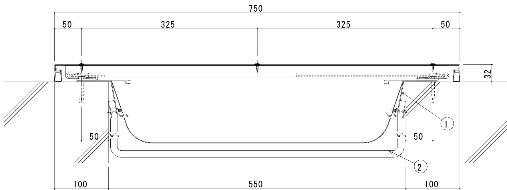
S550-EE (遮炎仕様) 断面図
