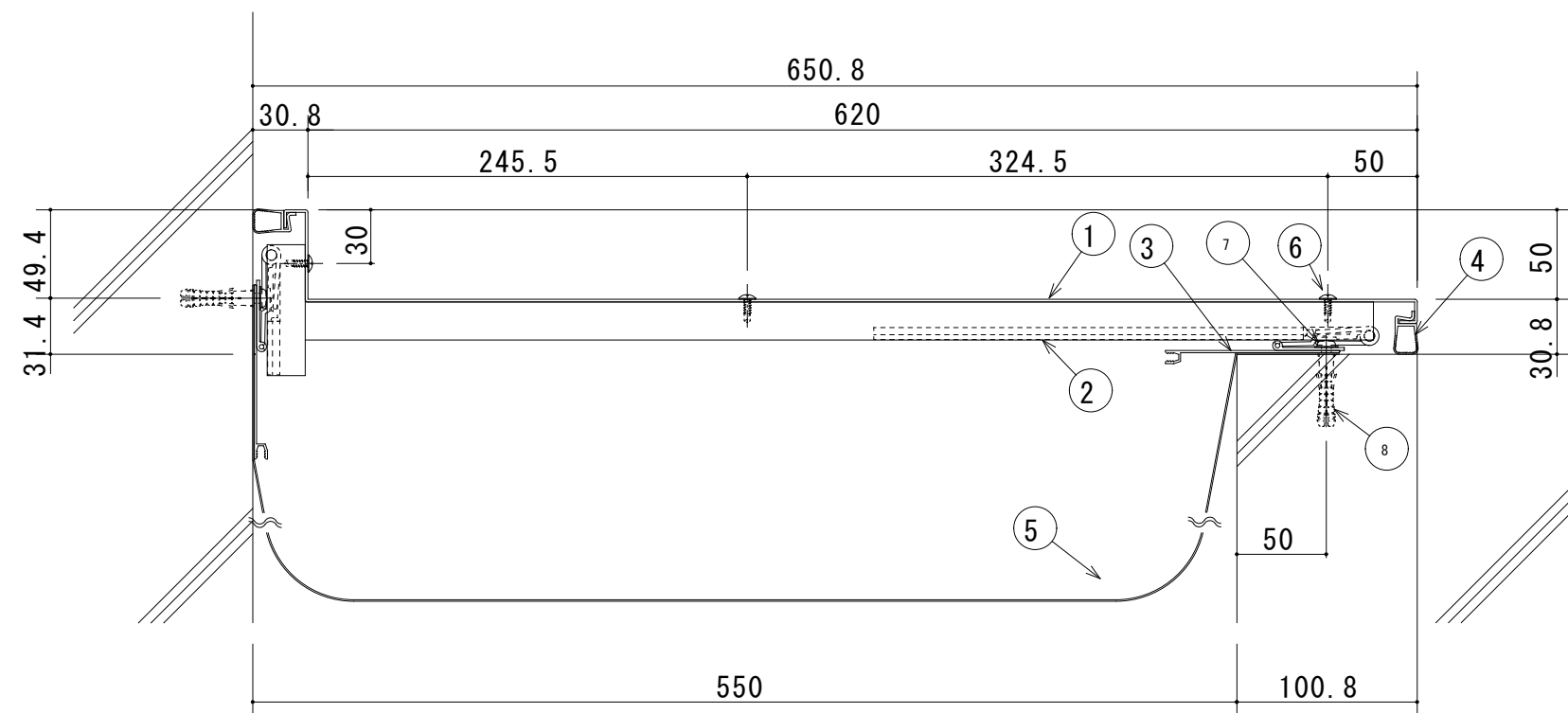
S550-ECE 断面図
