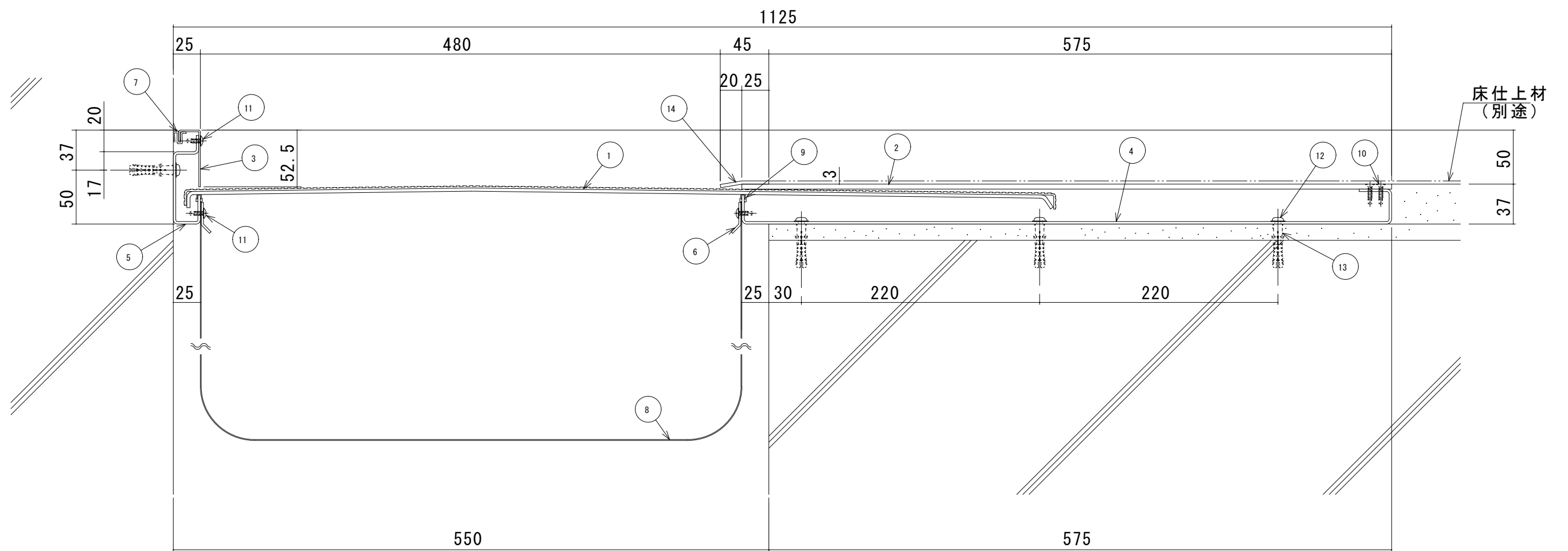
S550-FCHM 断面図
