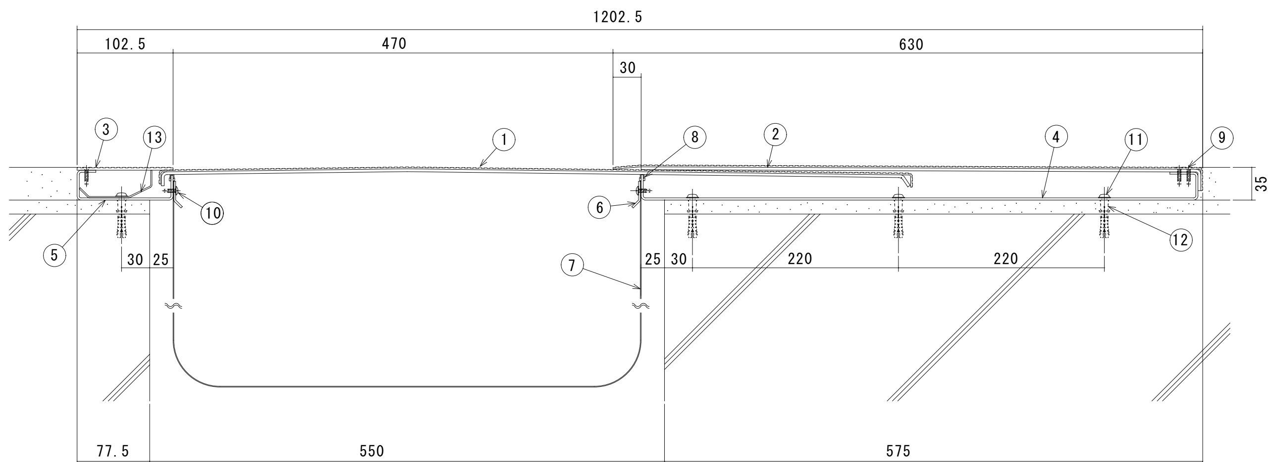
S550-FH-AS 断面図
