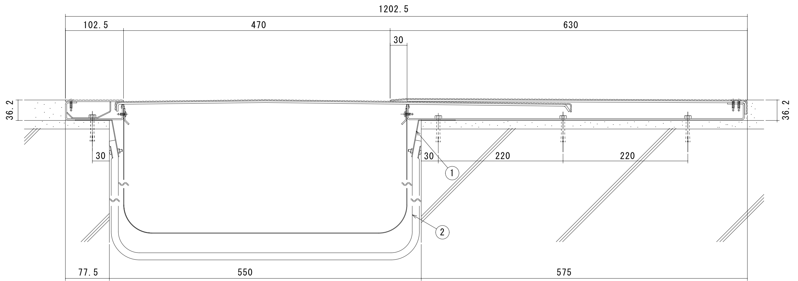
S550-FH-AS（遮炎仕様） 断面図
