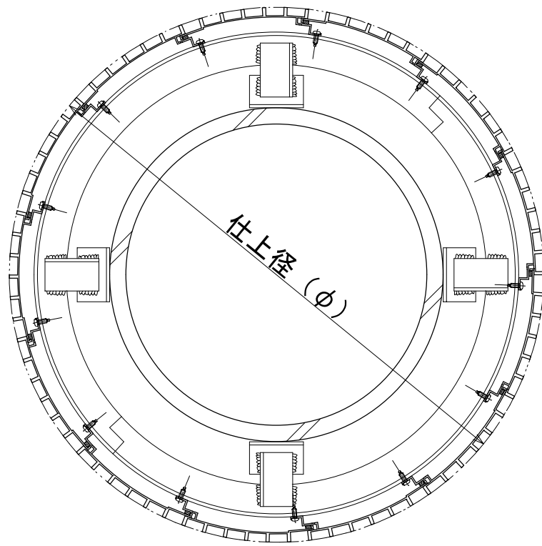
【平面参考納まり図】
