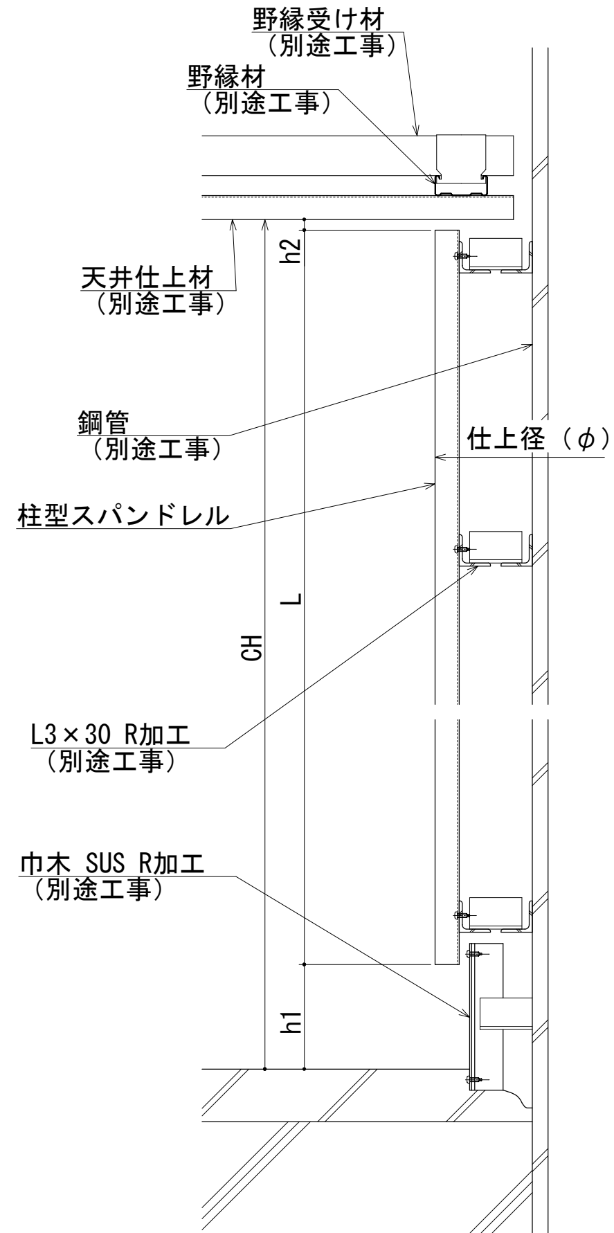
【縦断面参考納まり図】
