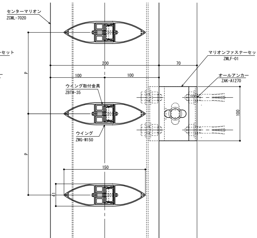
ウイング ZWG-W150
