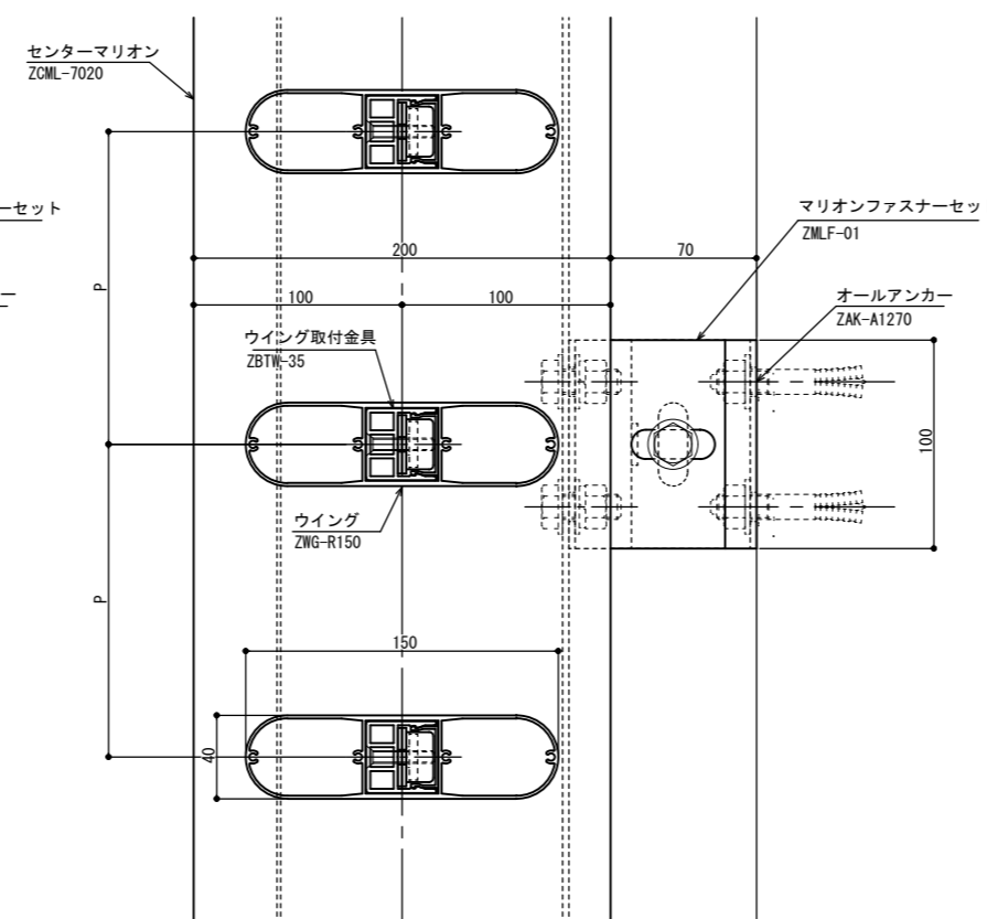
ウイング ZWG-R150
