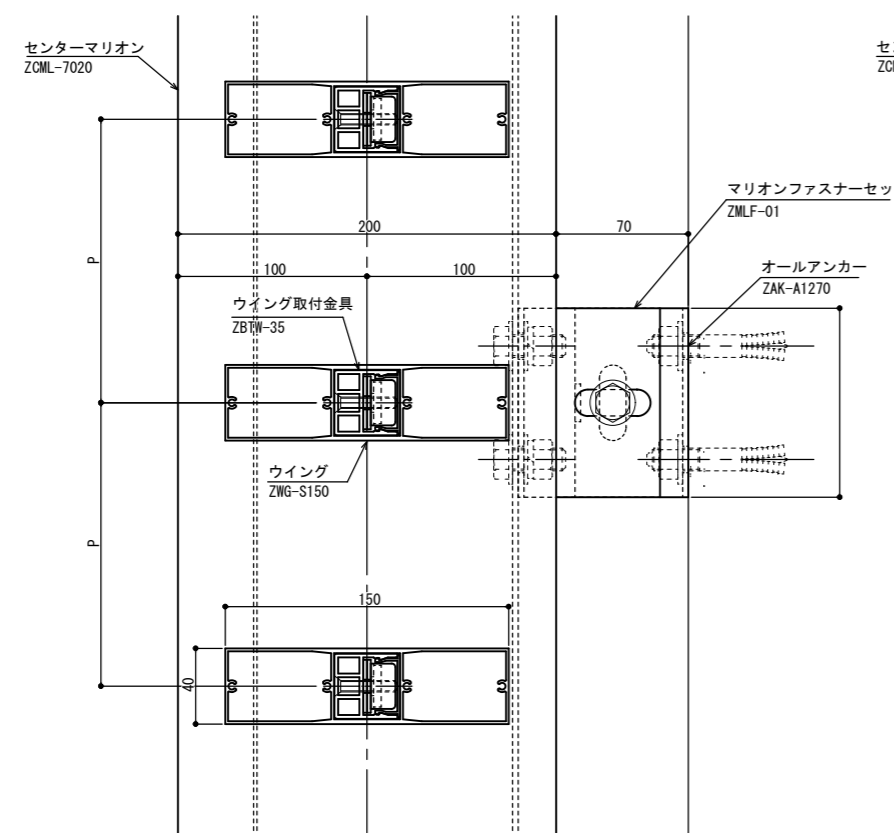
ウイング ZWG-S150
