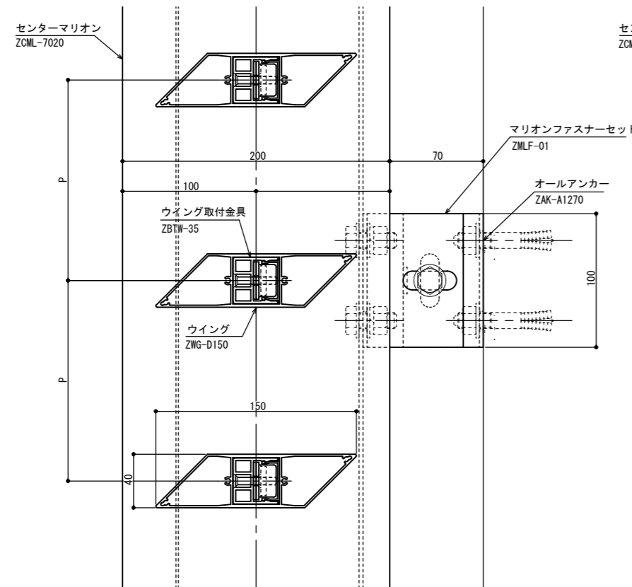
ウイング ZWG-D150
