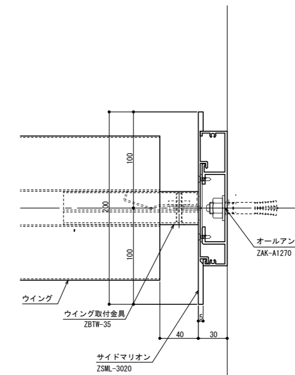
サイドマリオン ZSML-3020
