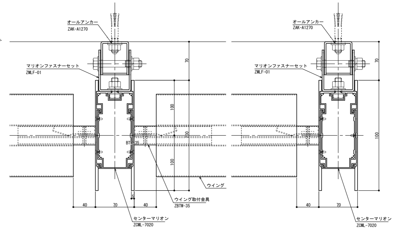
センターマリオン ZCML-7020
